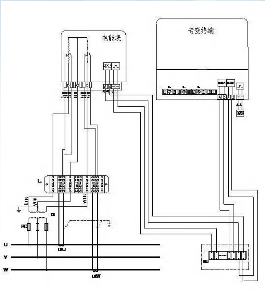
图 15 三相三线高压电能计量装置接线图
