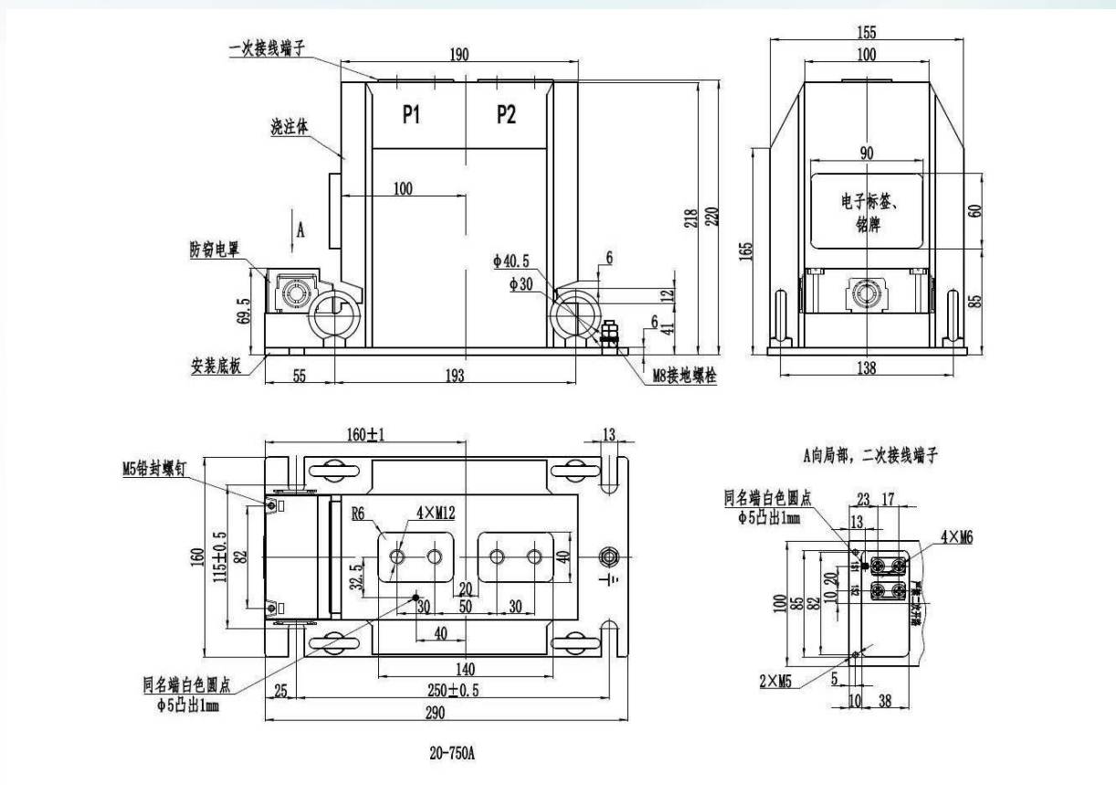
图 1 LJZN1-10、LJZN1-10G 型电流互感器外形尺寸 (mm)
