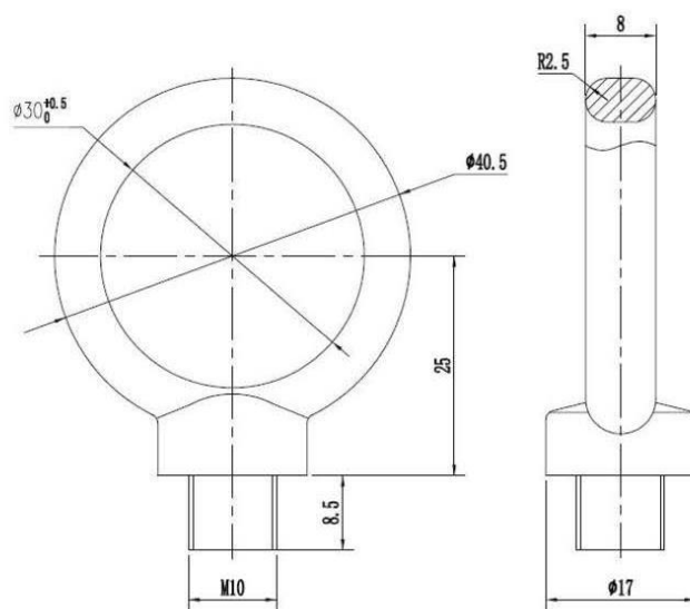
图 8 电流互感器吊环尺寸 (mm)
