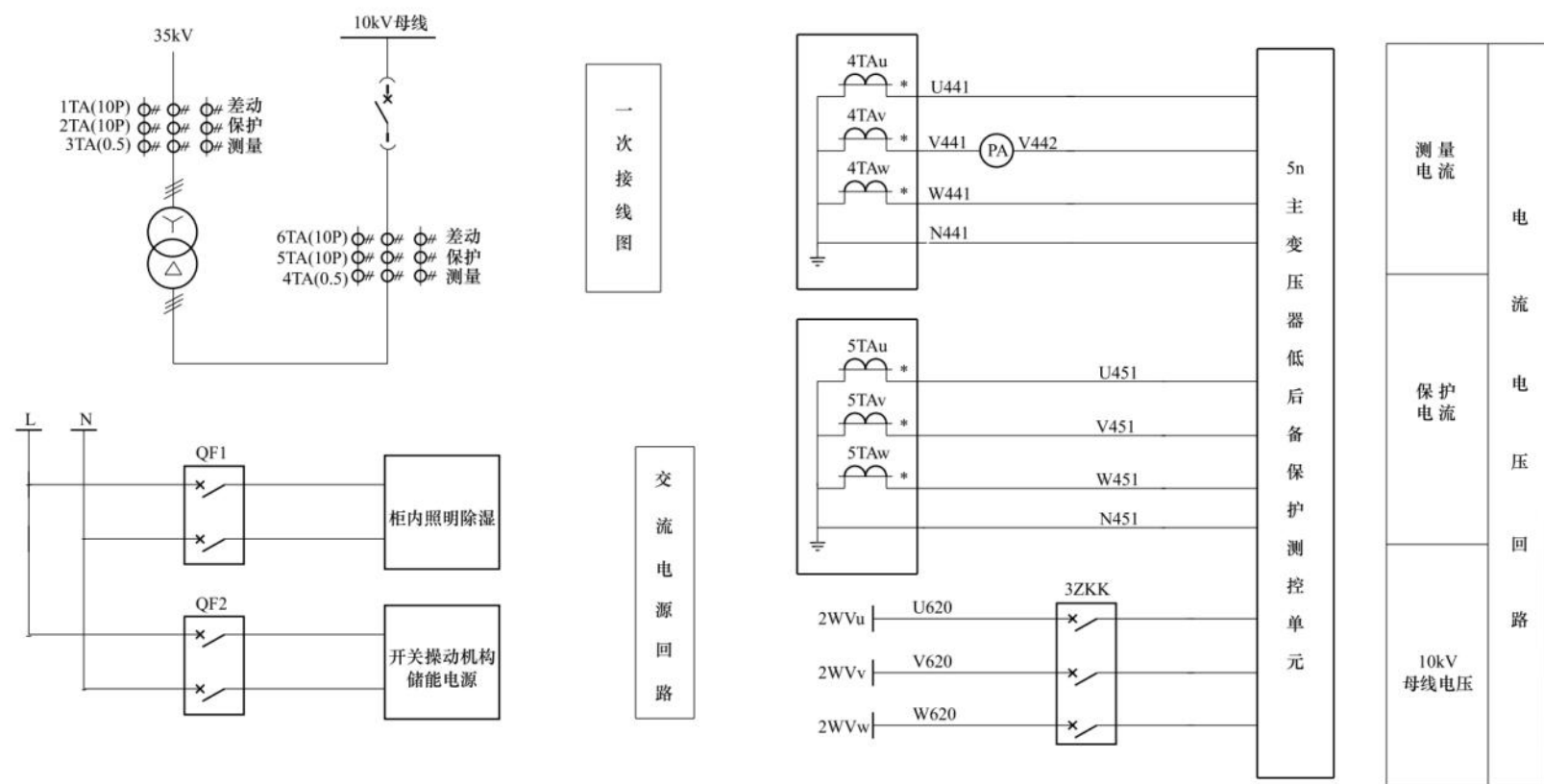
图 6-5 35kV 主变压器（差动保护）二次图——主变压器电流、电压回路图（二）
