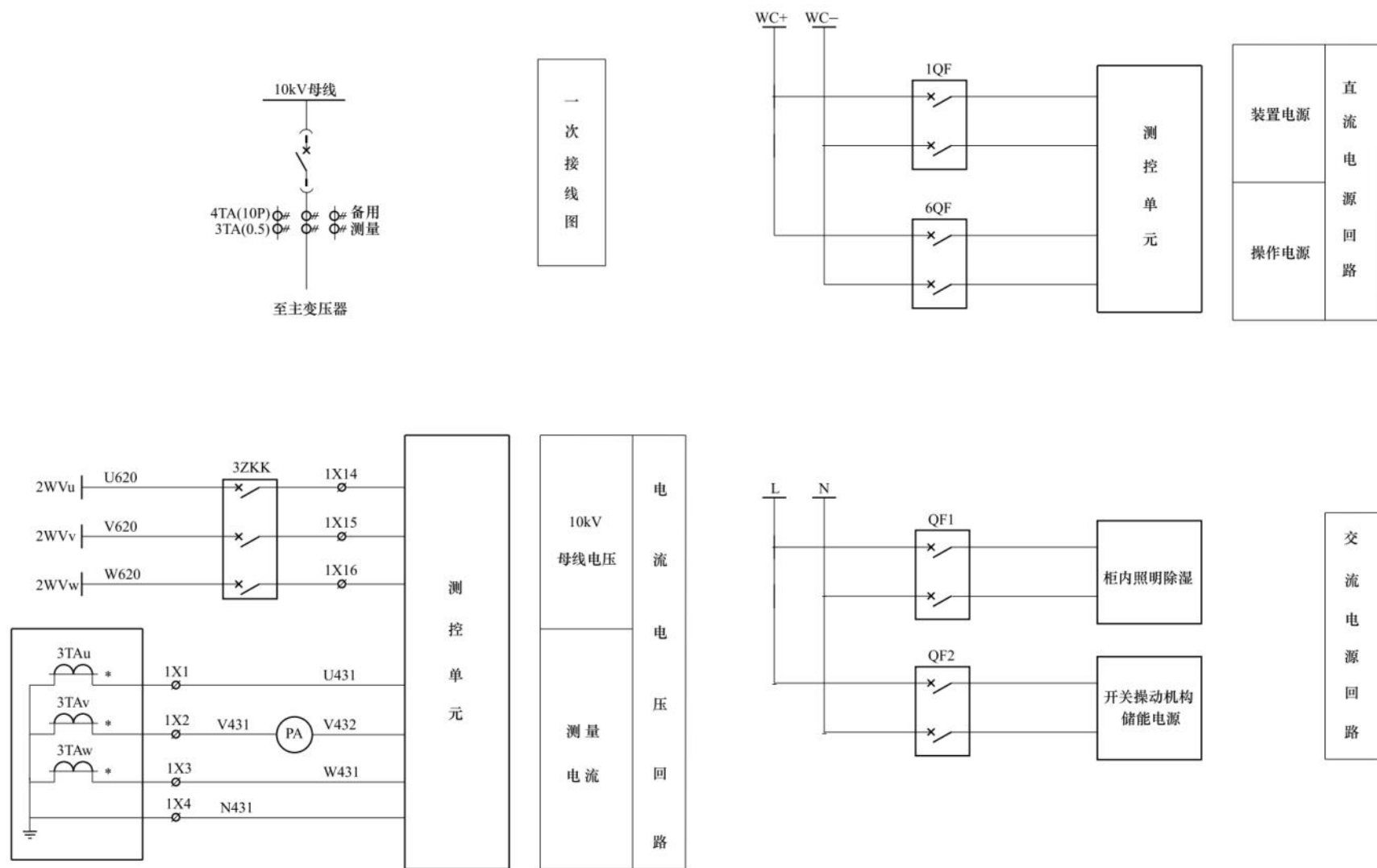
图 6-13 35kV 主变压器（电流保护）二次图——主变压器 10kV 次总开关电流电压回路图
