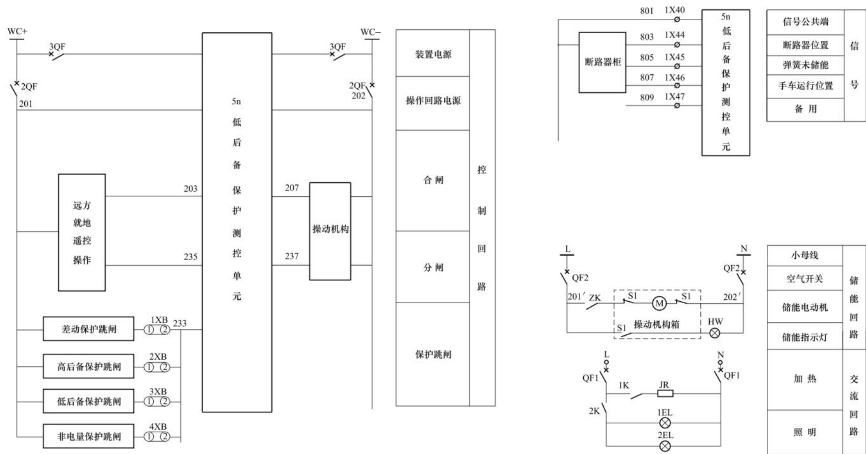
图 6-8 35kV 主变压器（差动保护）二次图——主变压器 10kV 侧开关控制信号回路图
