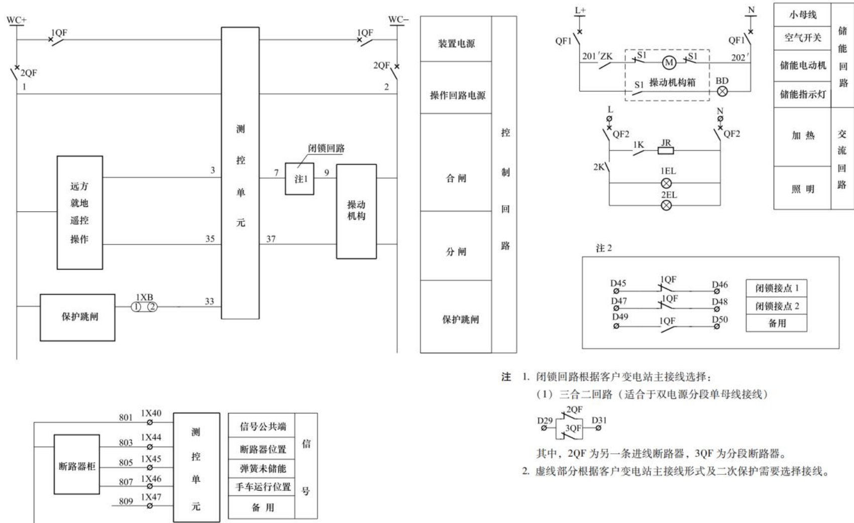
图 6-16 10kV 电源进线控制信号回路图
