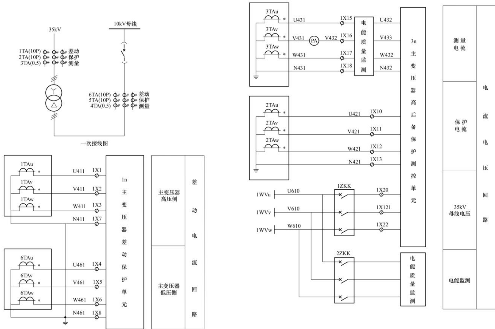
图 6-4 35kV 主变压器（差动保护）二次图——主变压器电流、电压回路图（一）
