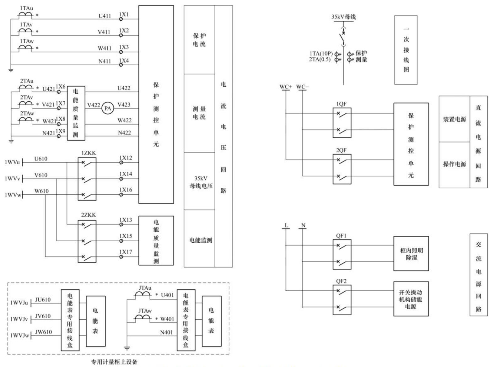
图 6-1 35kV 进线保护二次图——35kV 进线电流电压回路图
