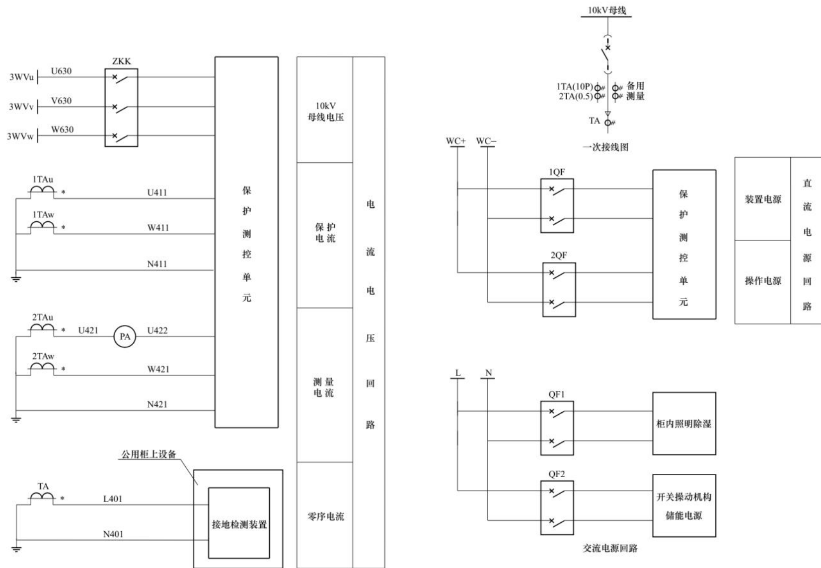
图 6-17 10kV 出线电流电压回路图
