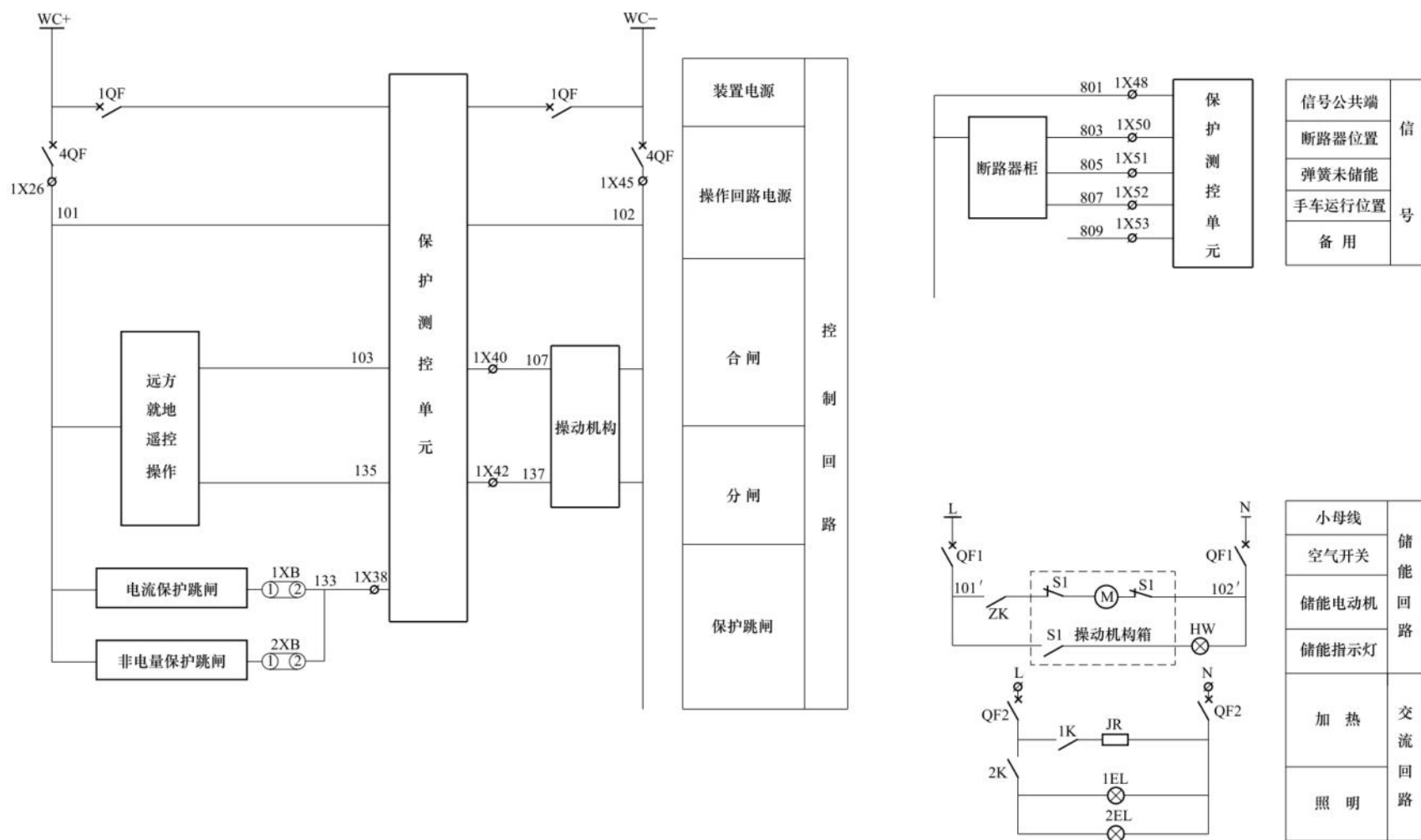
图 6-12 35kV 主变压器（电流保护）二次图——主变压器 35kV 侧开关控制信号回路图
