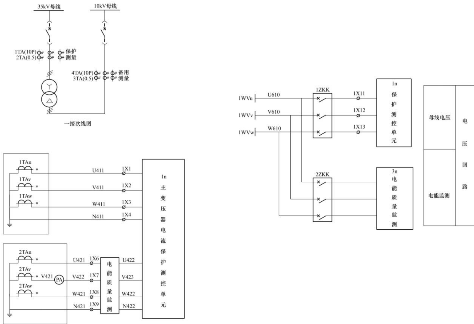
图 6-10 35kV 主变压器（电流保护）二次图——主变压器高压侧电流、电压回路图
