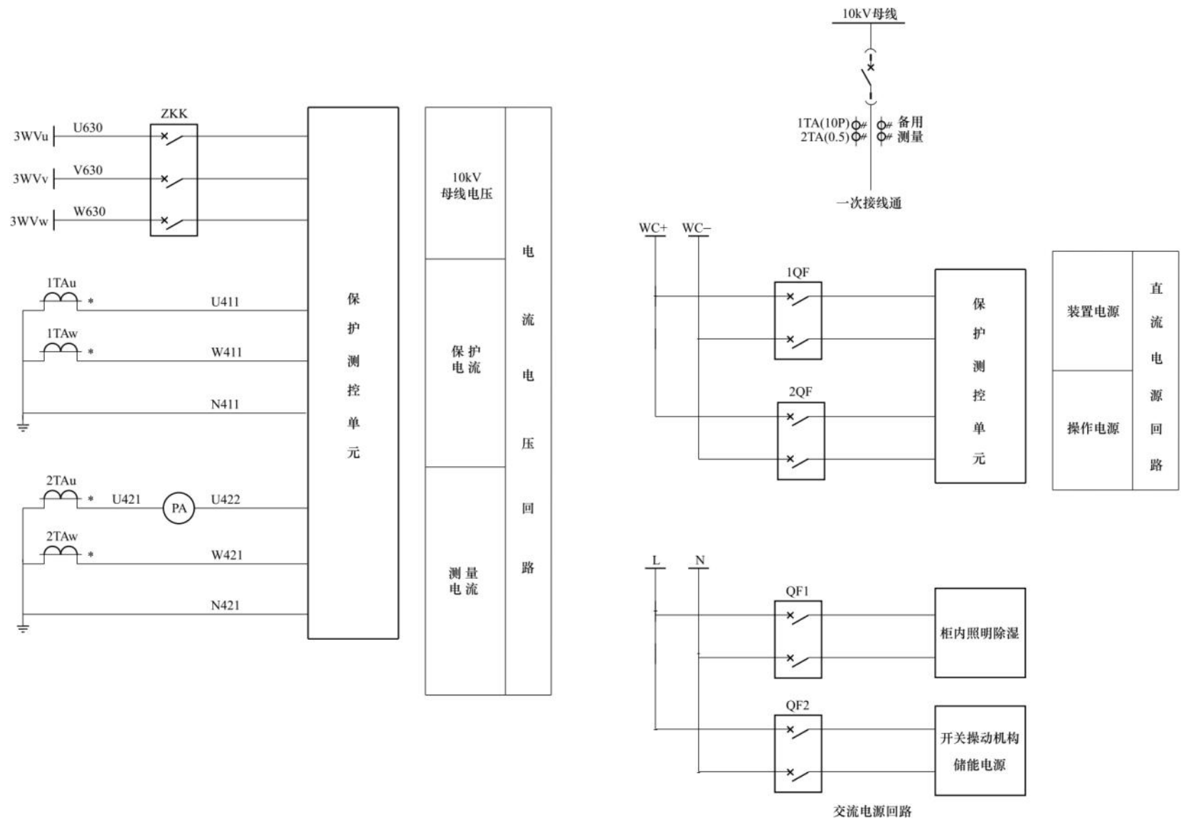
图 6-15 10kV 电源进线电流电压回路图
