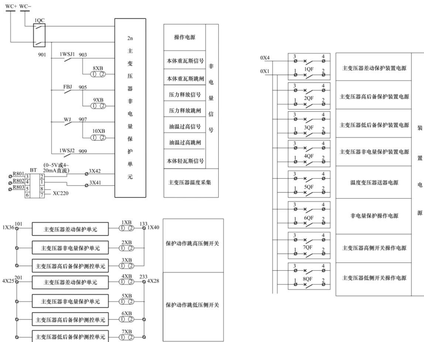
图 6-6 35kV 主变压器（差动保护）二次图——主变压器非电量保护及主变压器保护屏电源回路图
