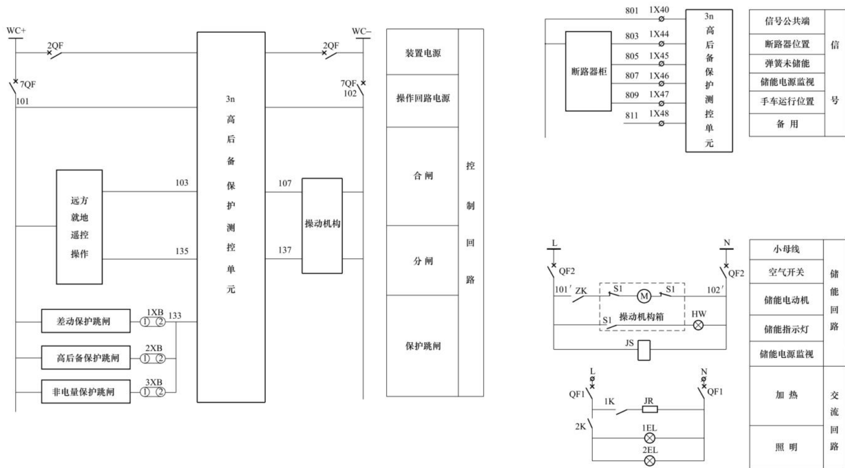
图 6-7 35kV 主变压器（差动保护）二次图——主变压器 35kV 侧开关控制信号回路图
