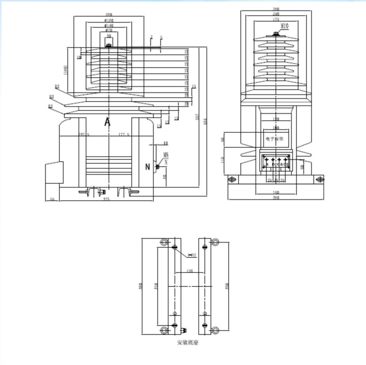
图 12 JDZXW-35 型接地式电压互感器外形尺寸 (mm)
