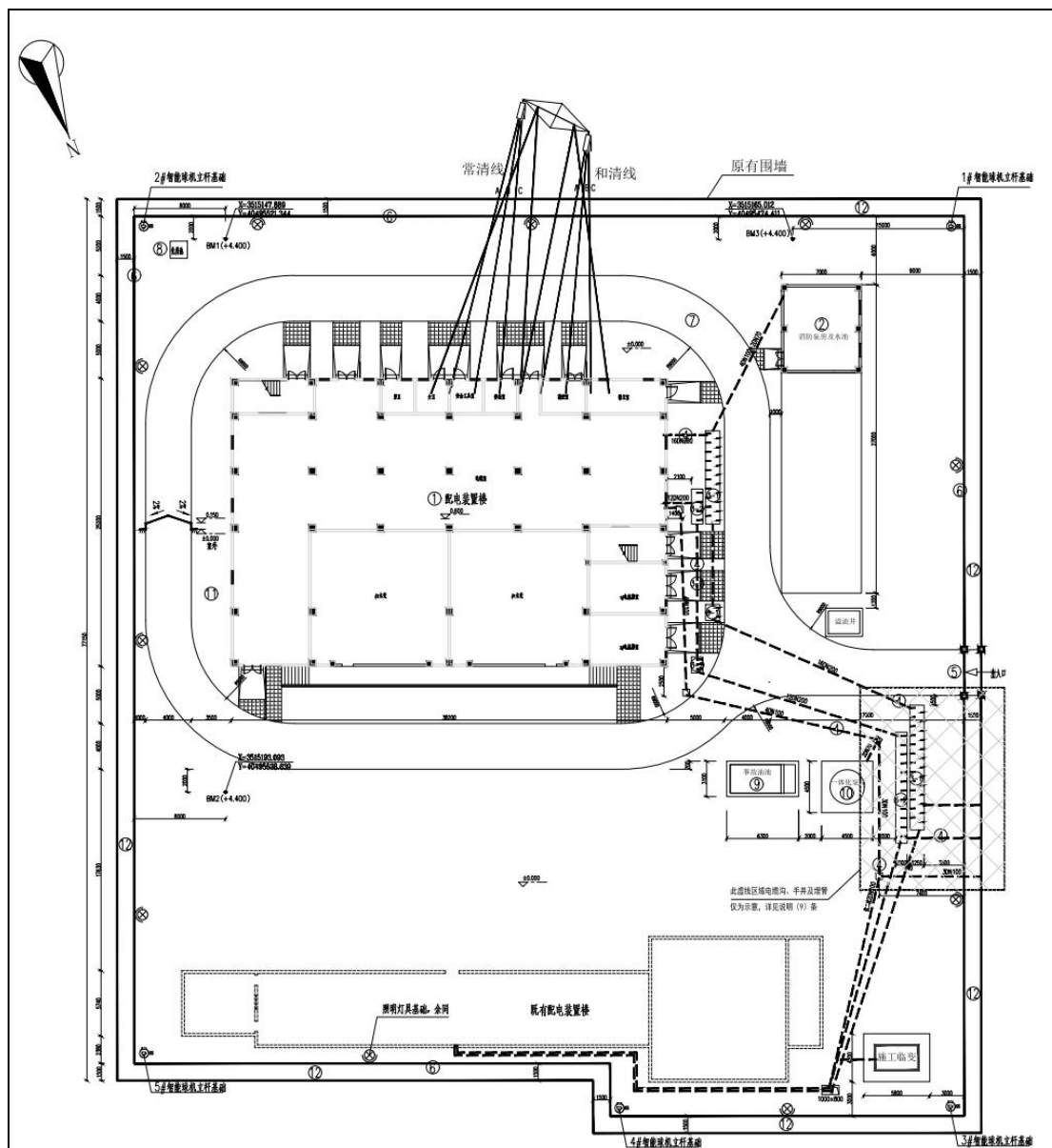
图 1-1 清凉 110 千伏变电站总平面布置图
