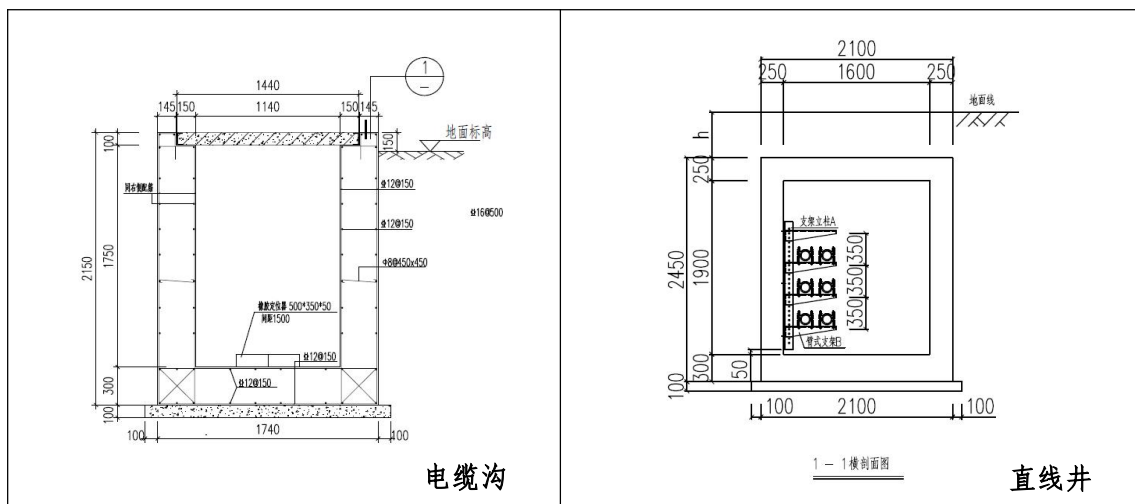
图 1.1-4 新建电缆断面图
