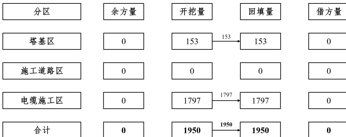
图 1.1-5 土石方平衡流向框图 单位：m 3
