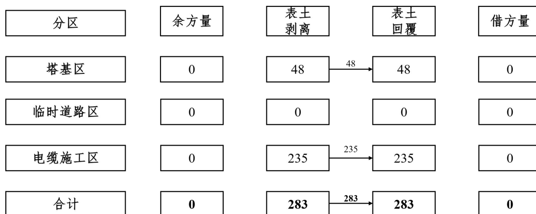
图 1.1-6 表土平衡流向框图 单位: m 3
