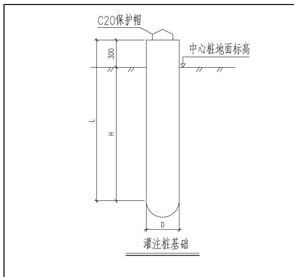
图 1.1-3 本工程塔基基础图
