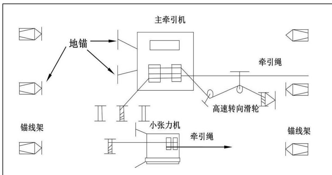
图 1.1-5 牵引场布置形式示意图
