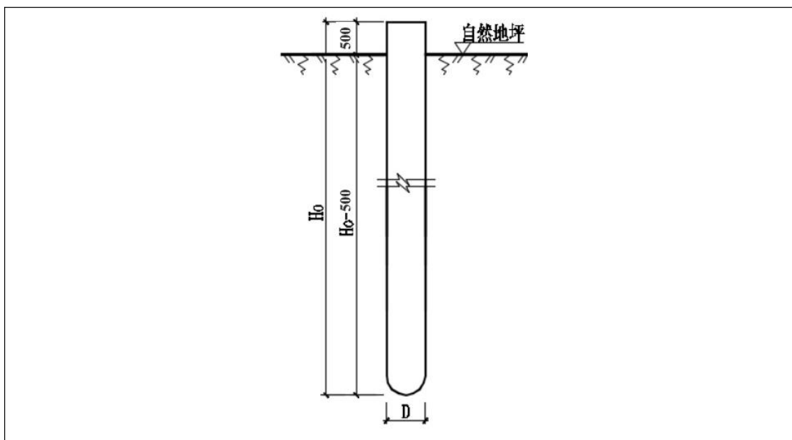
图 1.1-3 单桩灌注桩基础
