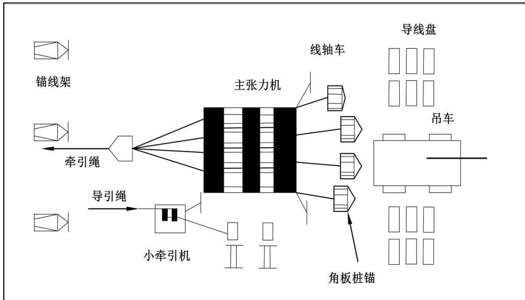
图 1.1-6 张力场布置形式示意图
