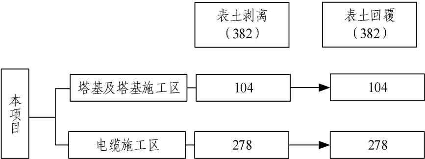
图 1.1-10 表土平衡流向框图 (单位: m 3 )
