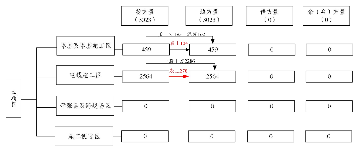
图 1.1-11 土石方挖填平衡流向框图（单位：m³）
