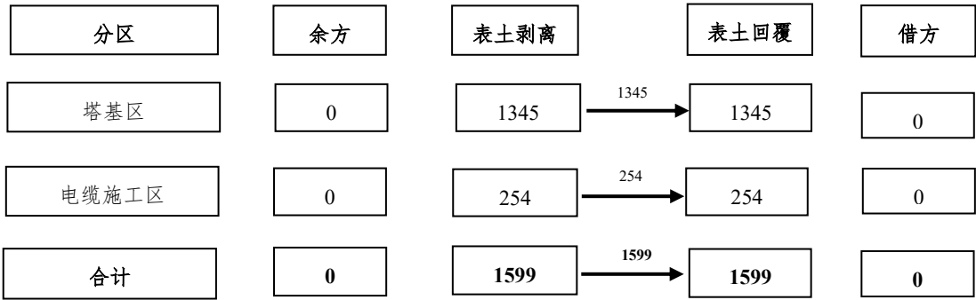
图 1.1-6 表土平衡流向框图 单位：m³
