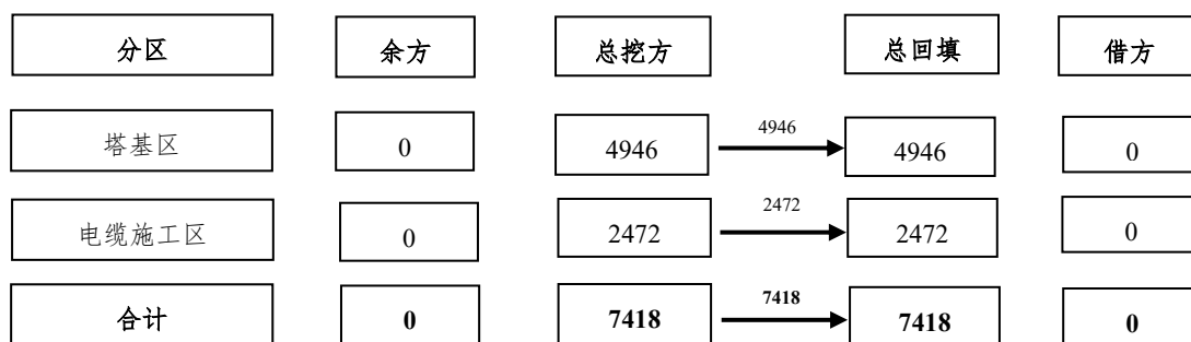
图 1.1-5 土石方平衡流向框图 单位：m 3
