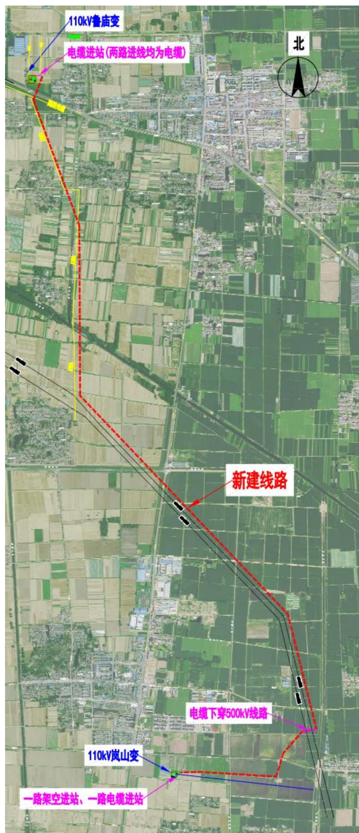
图 1.1-1 线路路径走向图
