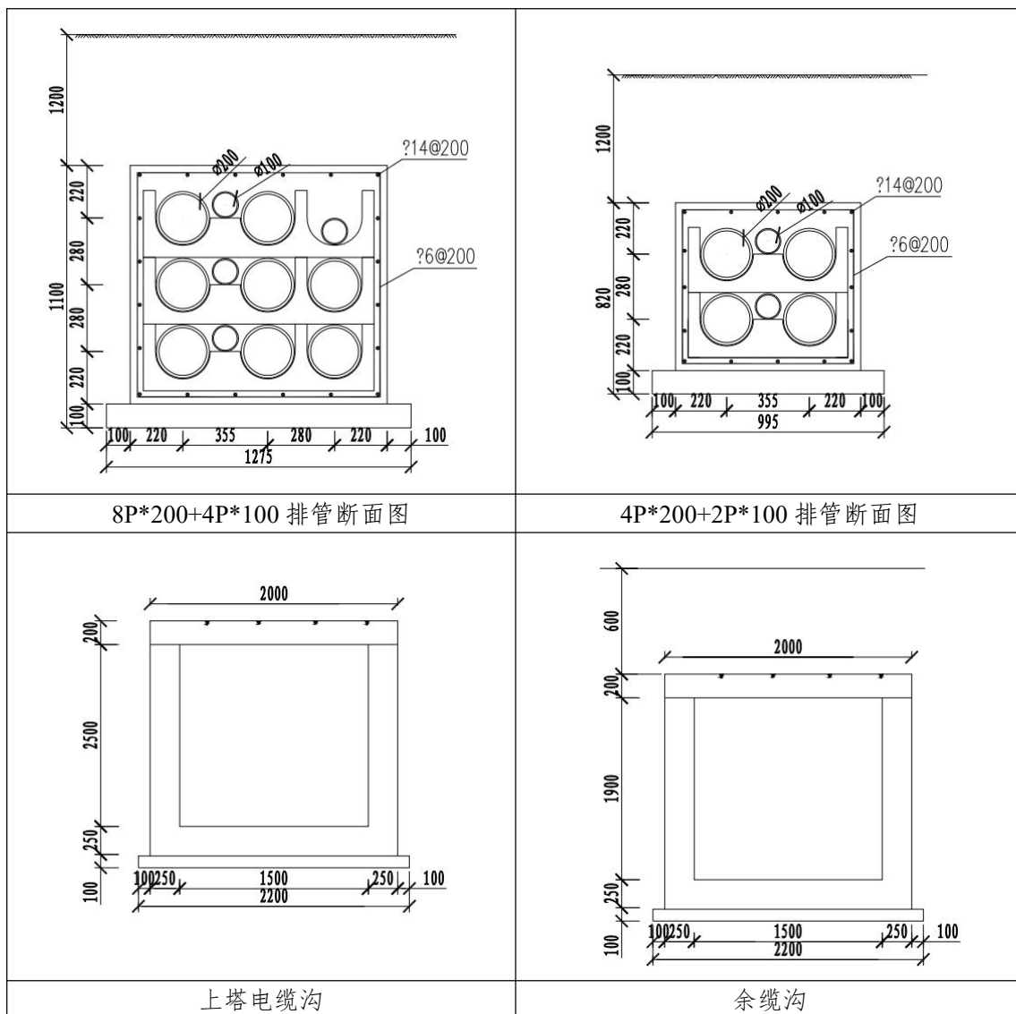
图 1.1-4 新建电缆断面图
