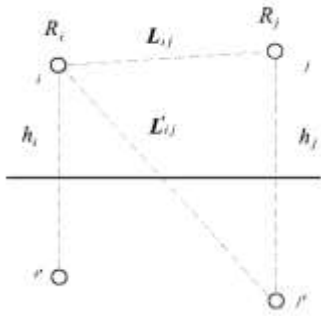
图 3.2-2 电位系数计算图
