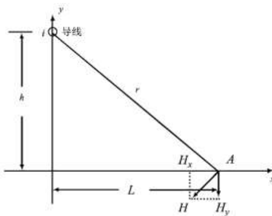
图 3.2-4 磁场向量图
