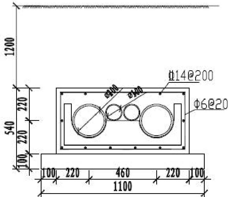
图 1-5 电缆排管断面图
