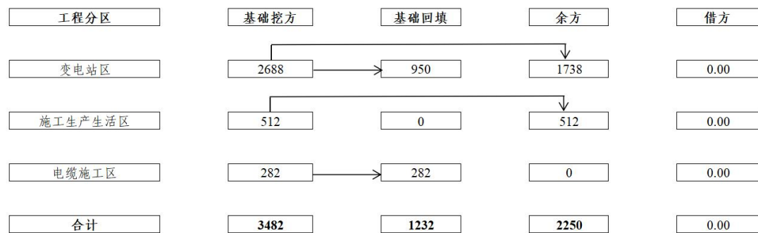
图 1-8 土石方平衡流向框图（单位：m 3 ）
