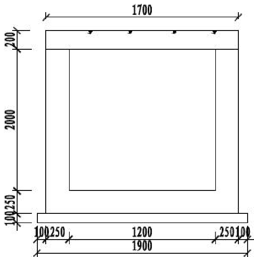
图 1-6 上塔电缆沟断面图
