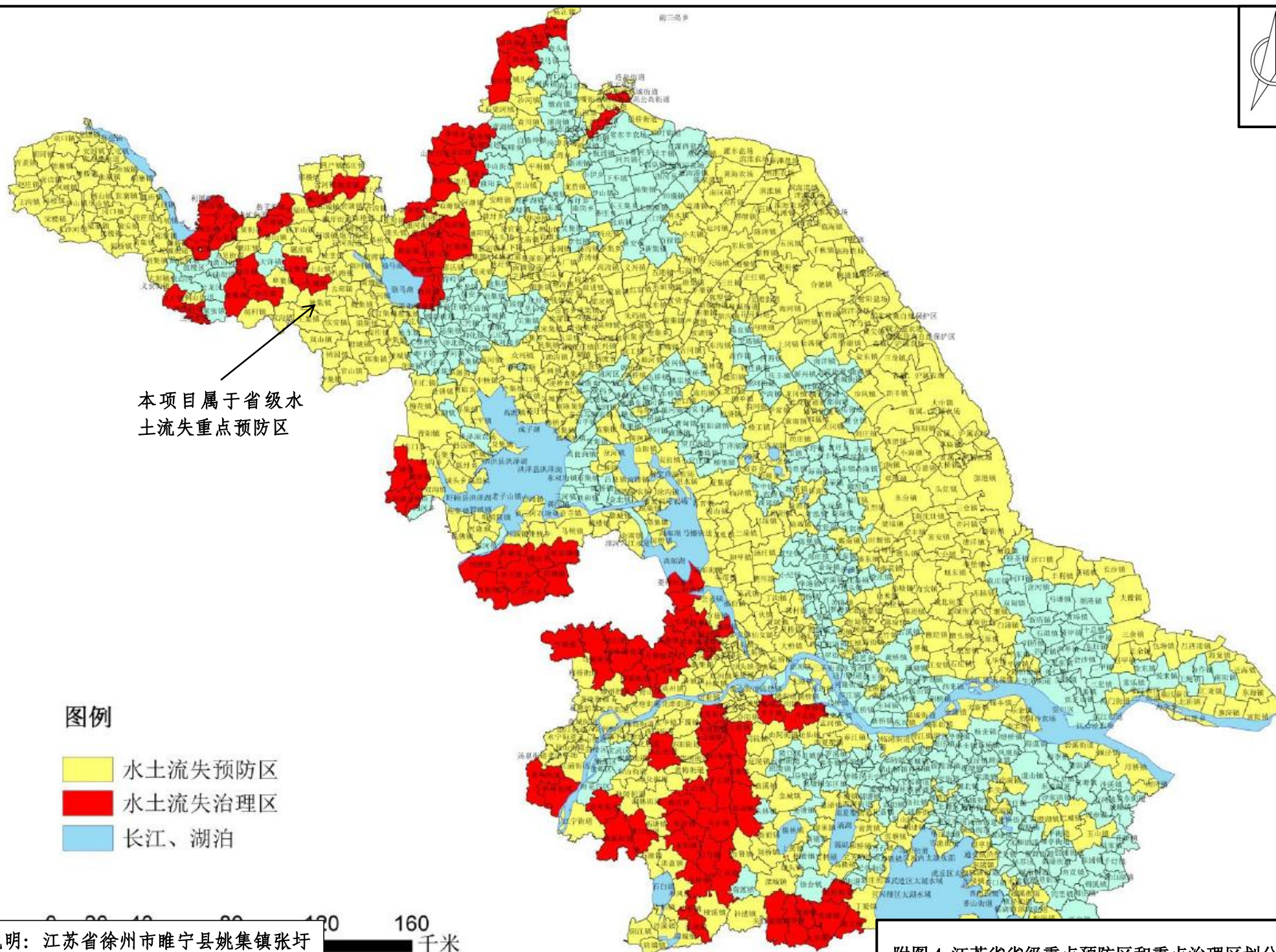
附图 4 江苏省省级重点预防区和重点治理区划分图
