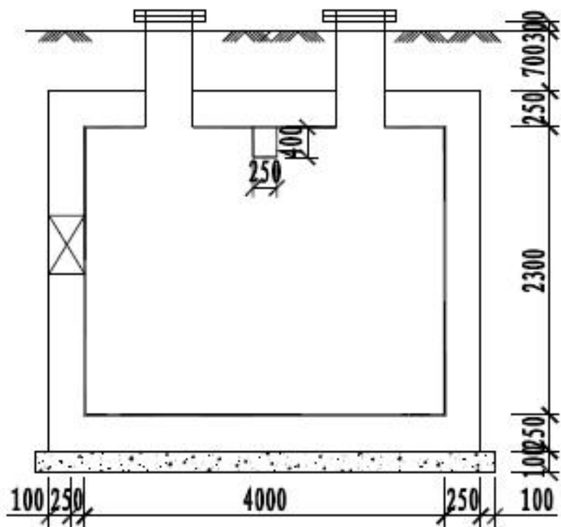
图 1-7 终端井断面图
