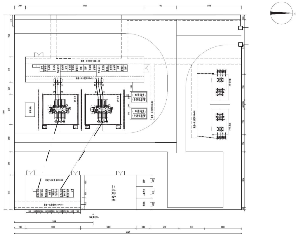
图 1-1 变电站平面布置图
