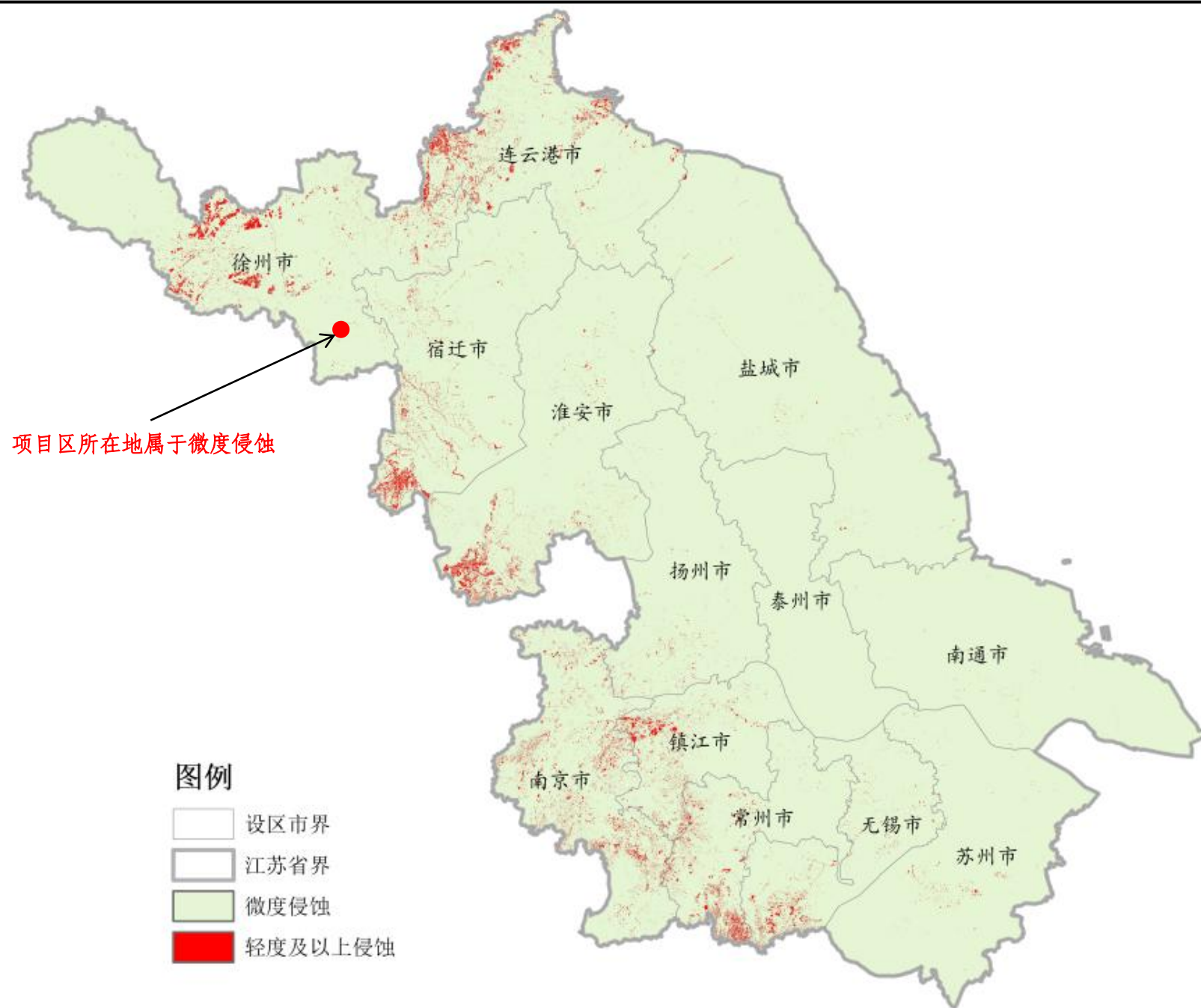
附图 3 项目区土壤侵蚀强度分布图
