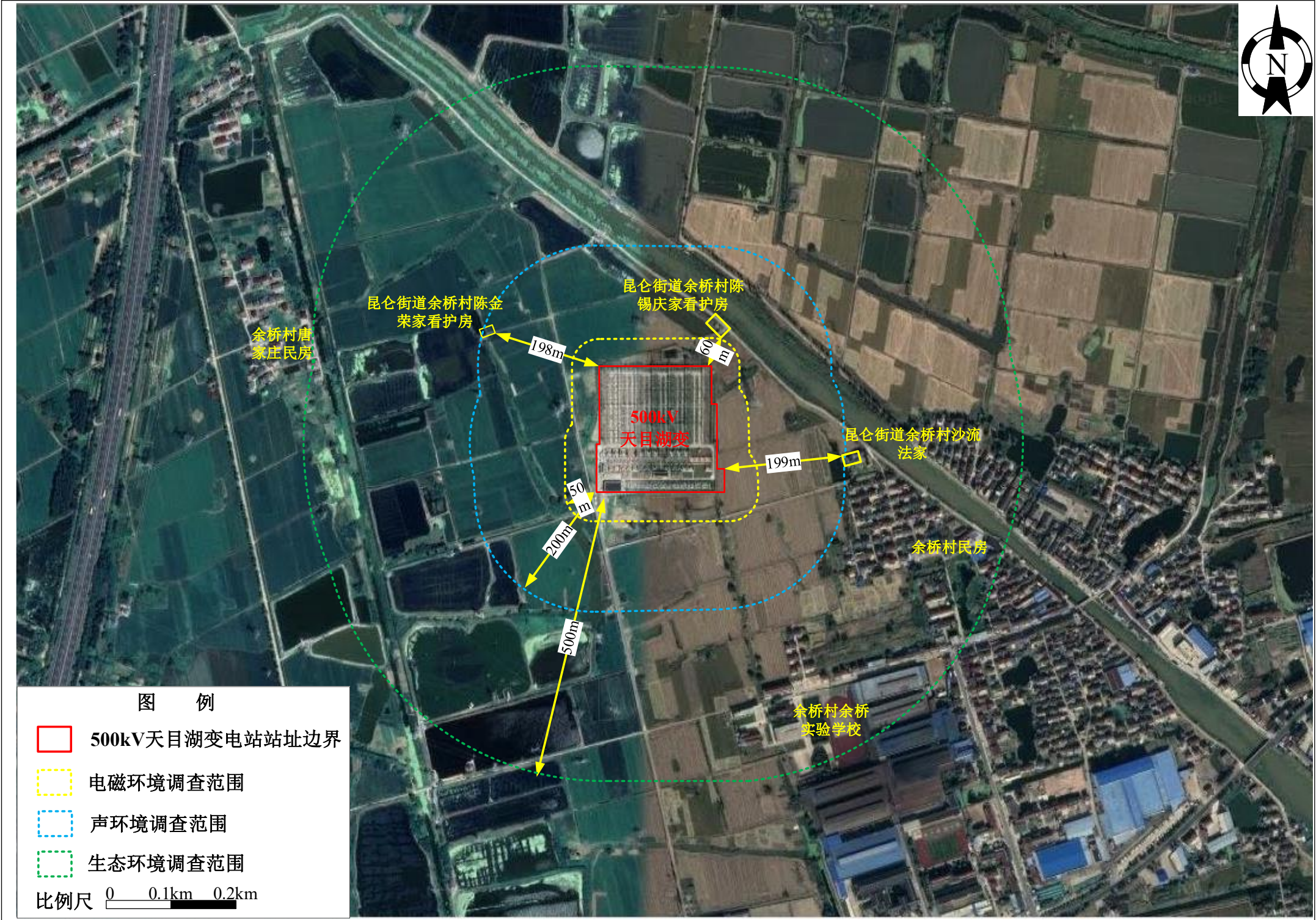
图 2-1 500kV 天目湖变电站周围环境示意图
