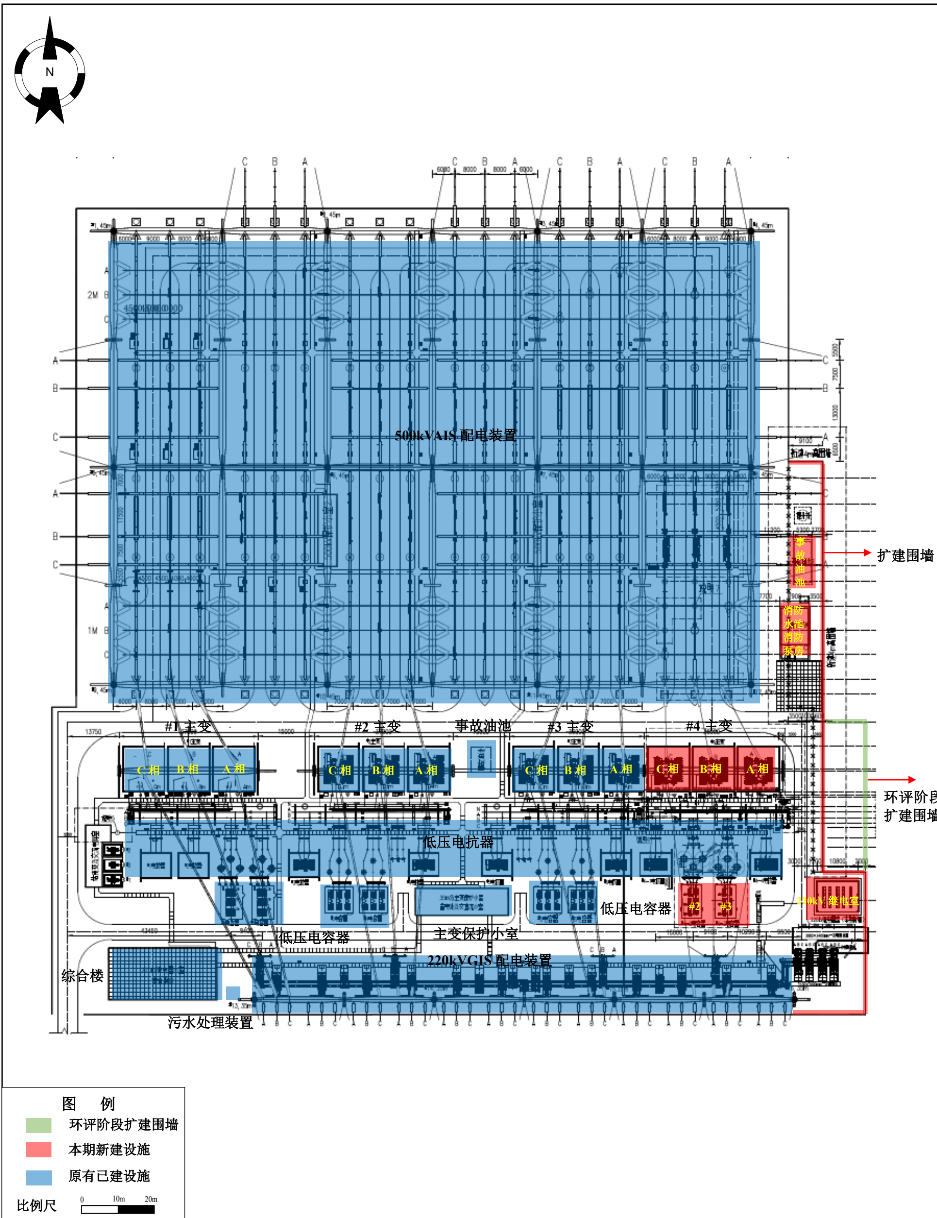
图 3-6 天目湖 500kV 变电站总平面布置图
