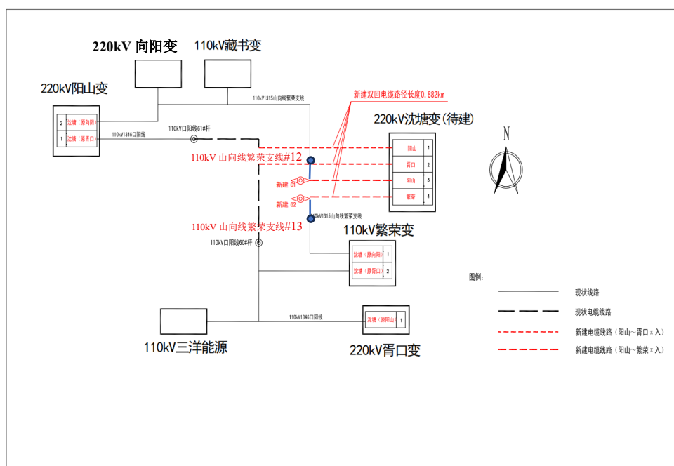
图 2-1 本项目实施后接线示意图
