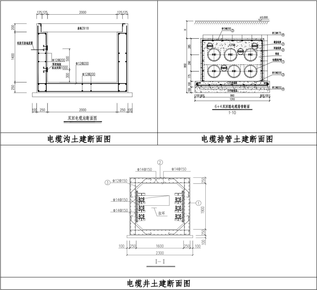
图 1.1-3 电缆土建断面图
