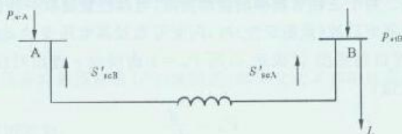
图 2 闪变传递计算示意
