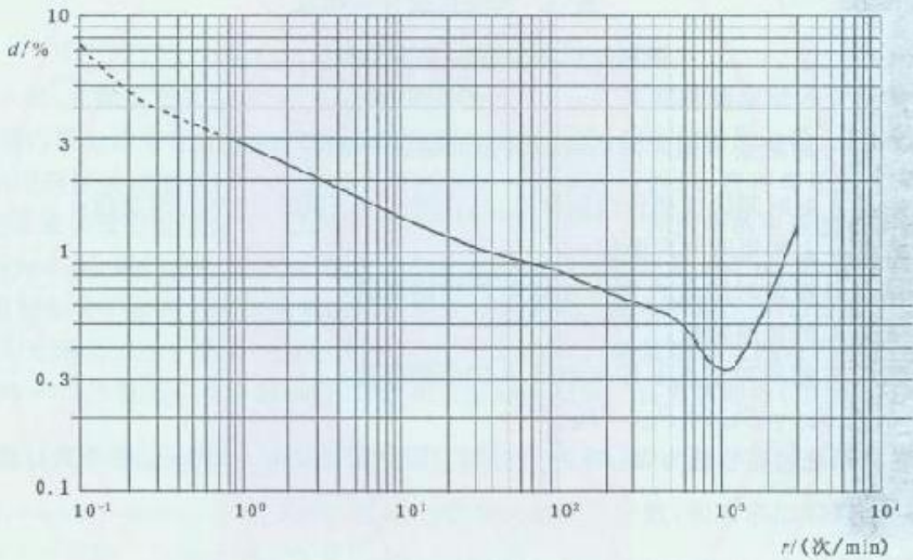
图 1 周期性矩形(或阶跃波)电压变动的单位闪变( P_{st}=1 )曲线 表 4 周期性矩形(或阶跃波)电压变动的单位闪变( P_{st}=1 )曲线对应数据
