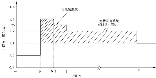
图 3 光伏发电系统高电压穿越要求
