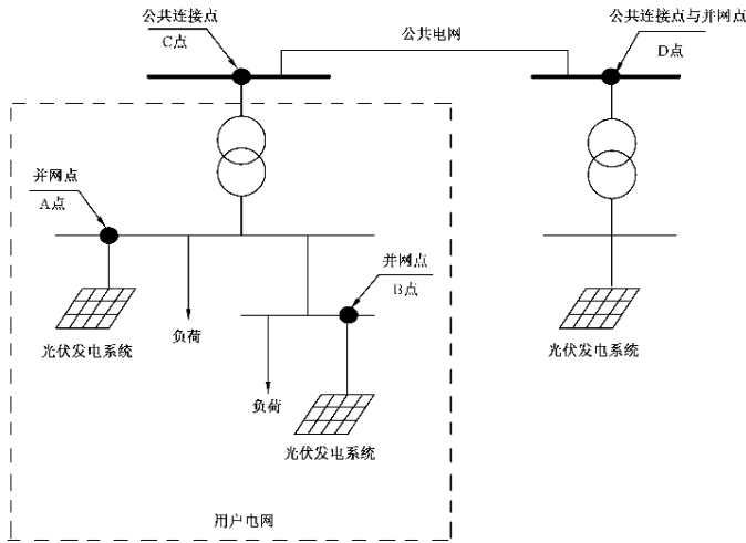
图 A.1 并网点和公共连接点示意图
