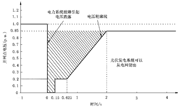
图 2 光伏发电系统低电压穿越要求
