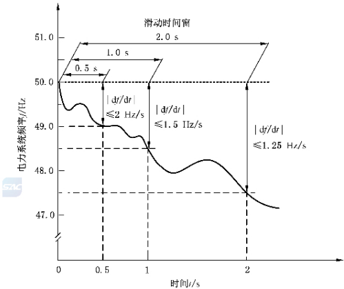
图 4 滑动时间窗与频率变化率示意图
