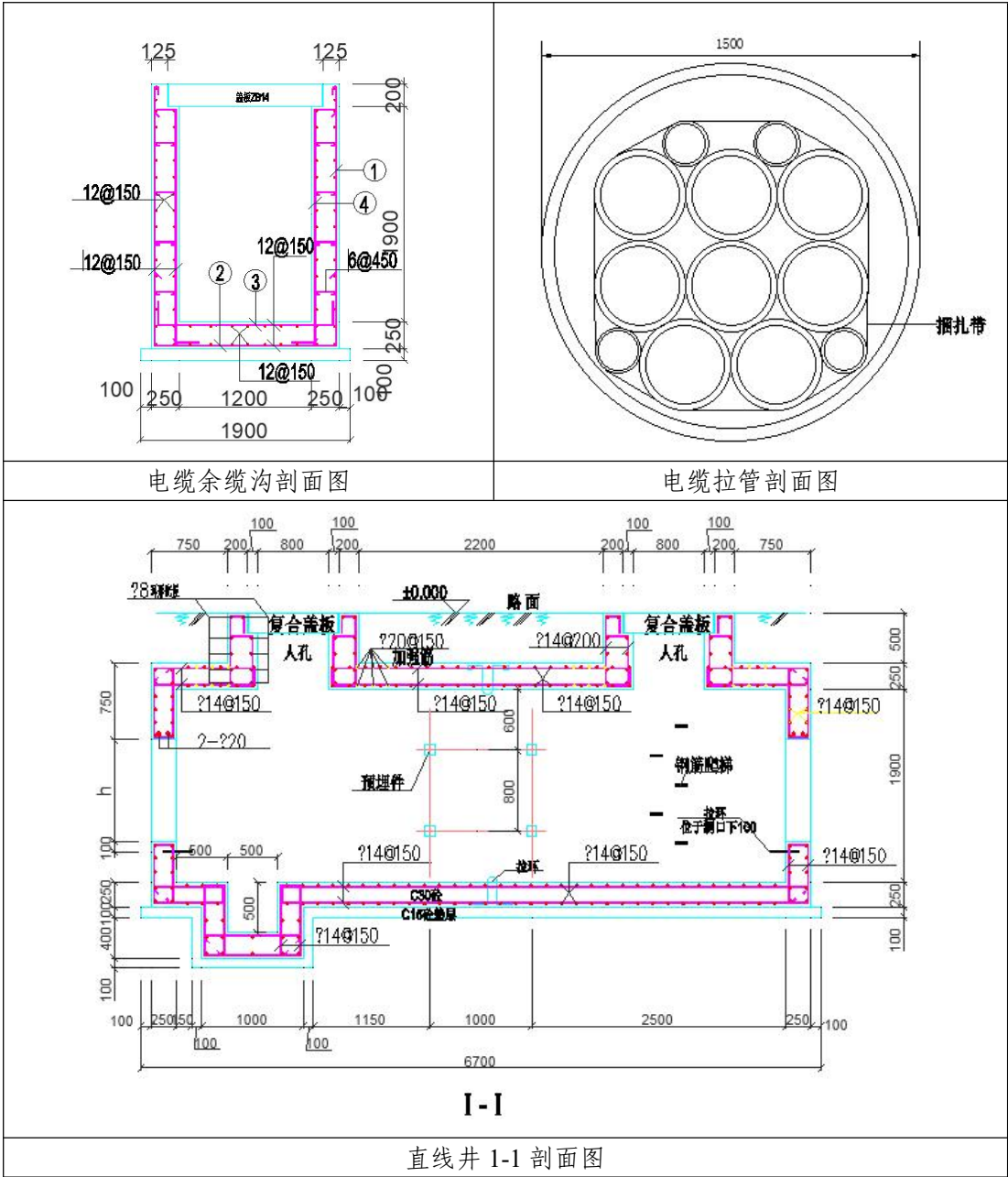
图 1.1-3 电缆拉管、沟及工作井剖面图
