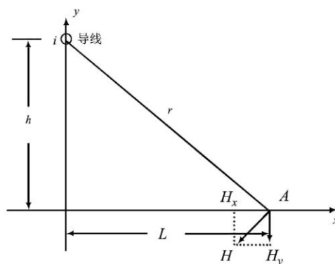
图 3.1-4 磁场向量图
