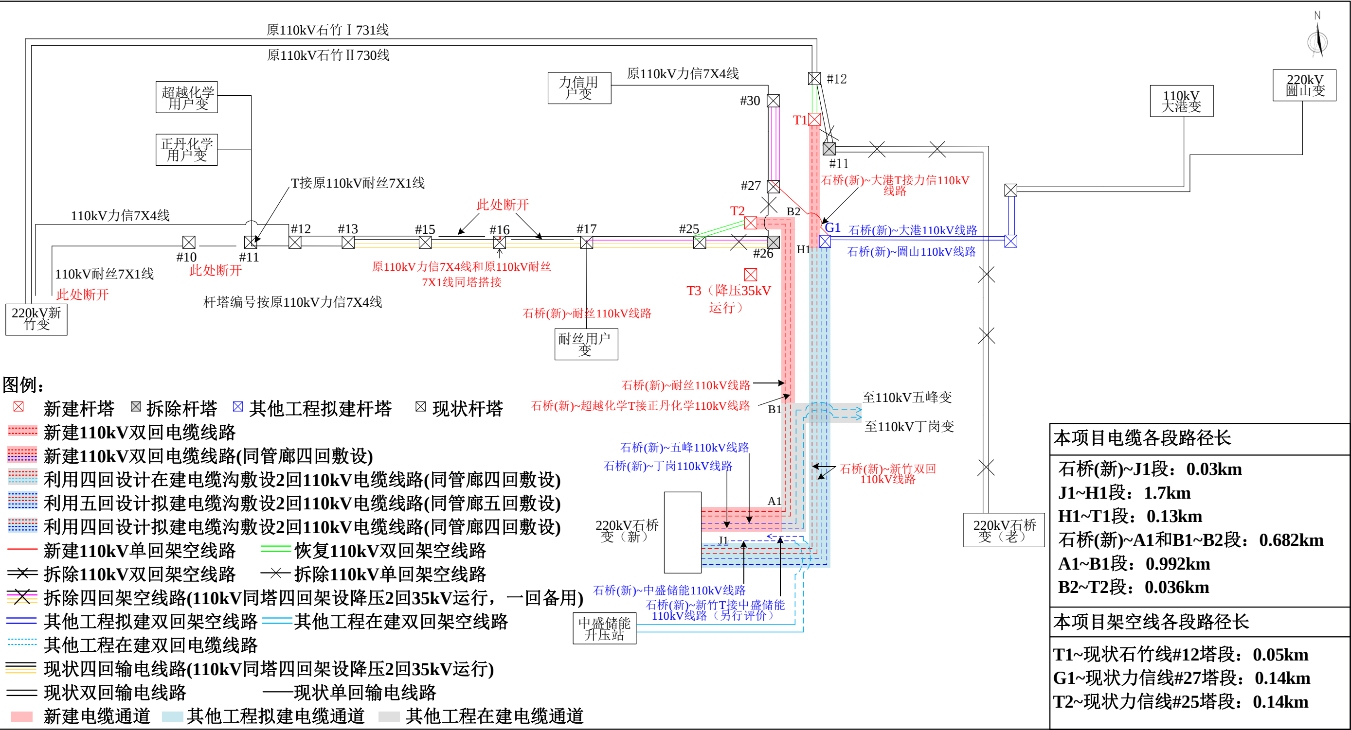
图 2-2 本项目实施后接线方案示意图
