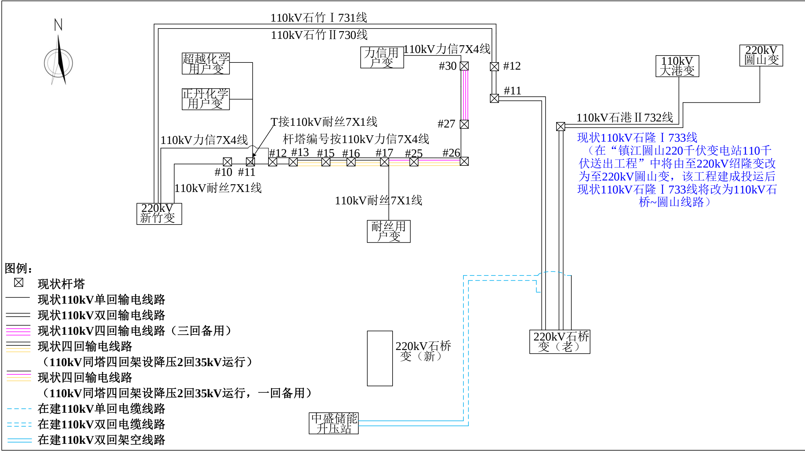
图 2-1 本项目实施前接线方案示意图
