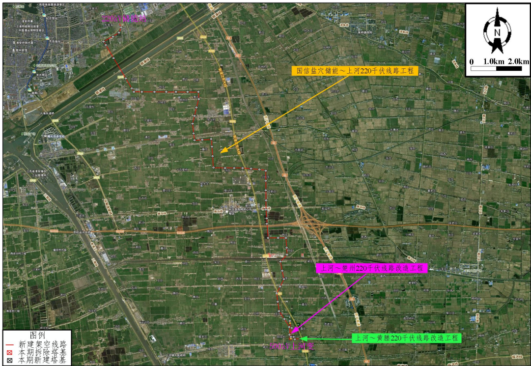
图 1.1-4 线路路径走向图
