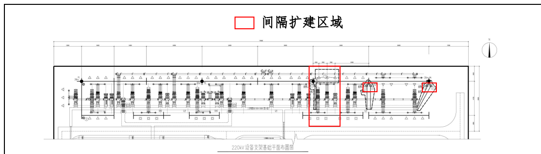
图 1.1-1 上河 500 千伏变电站 220 千伏间隔扩建工程平面布置图
