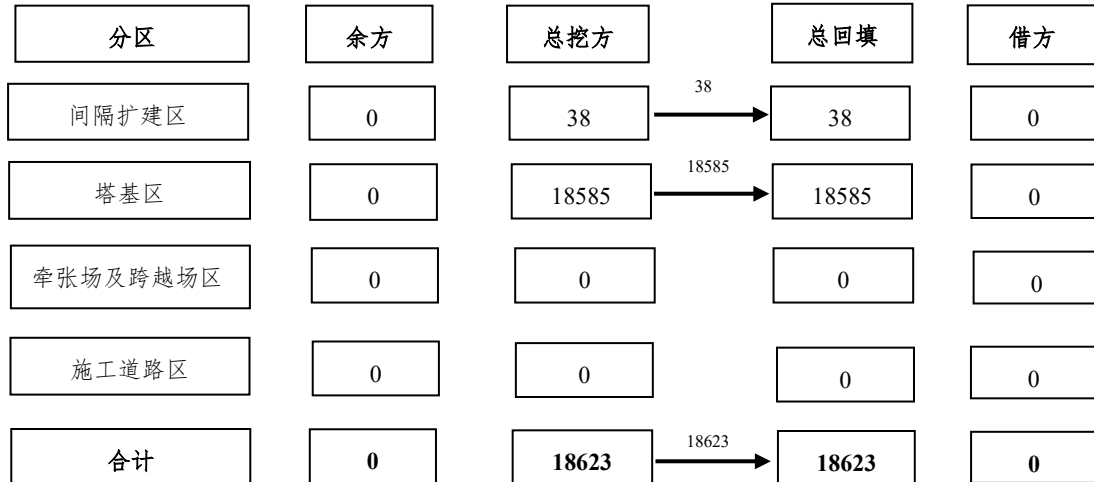
图 1.1-8 土石方平衡流向框图 单位：m 3
