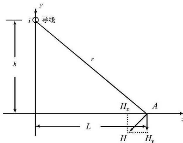
图 3.1-4 磁场向量图
