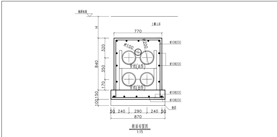
图 1.1-6 排管土建断面图
