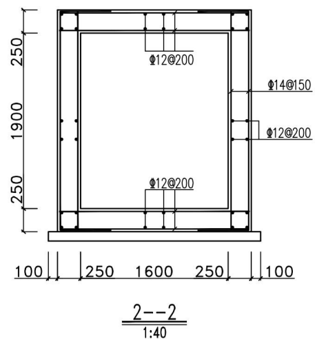
图 1.1-5 电缆井土建断面图
