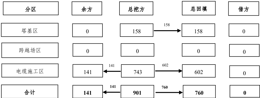
图 1.1-7 土石方平衡流向框图 单位：m³
