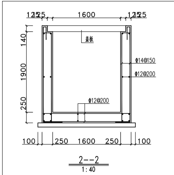
图 1.1-4 电缆沟土建断面图
