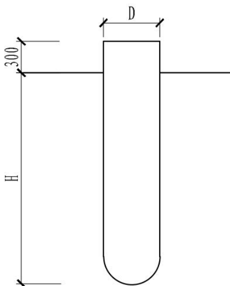
图 1-3 灌注桩基础示意图
