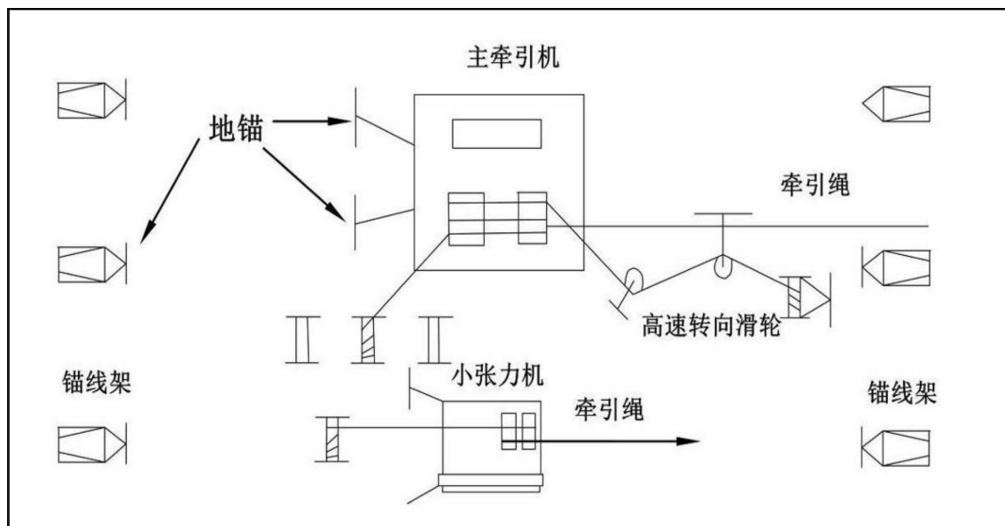
图1-6 牵引场布置示意图
