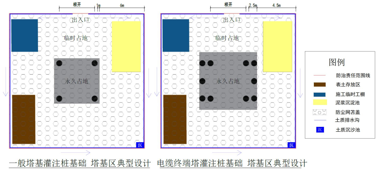
图 1-9 塔基区布置示意图
