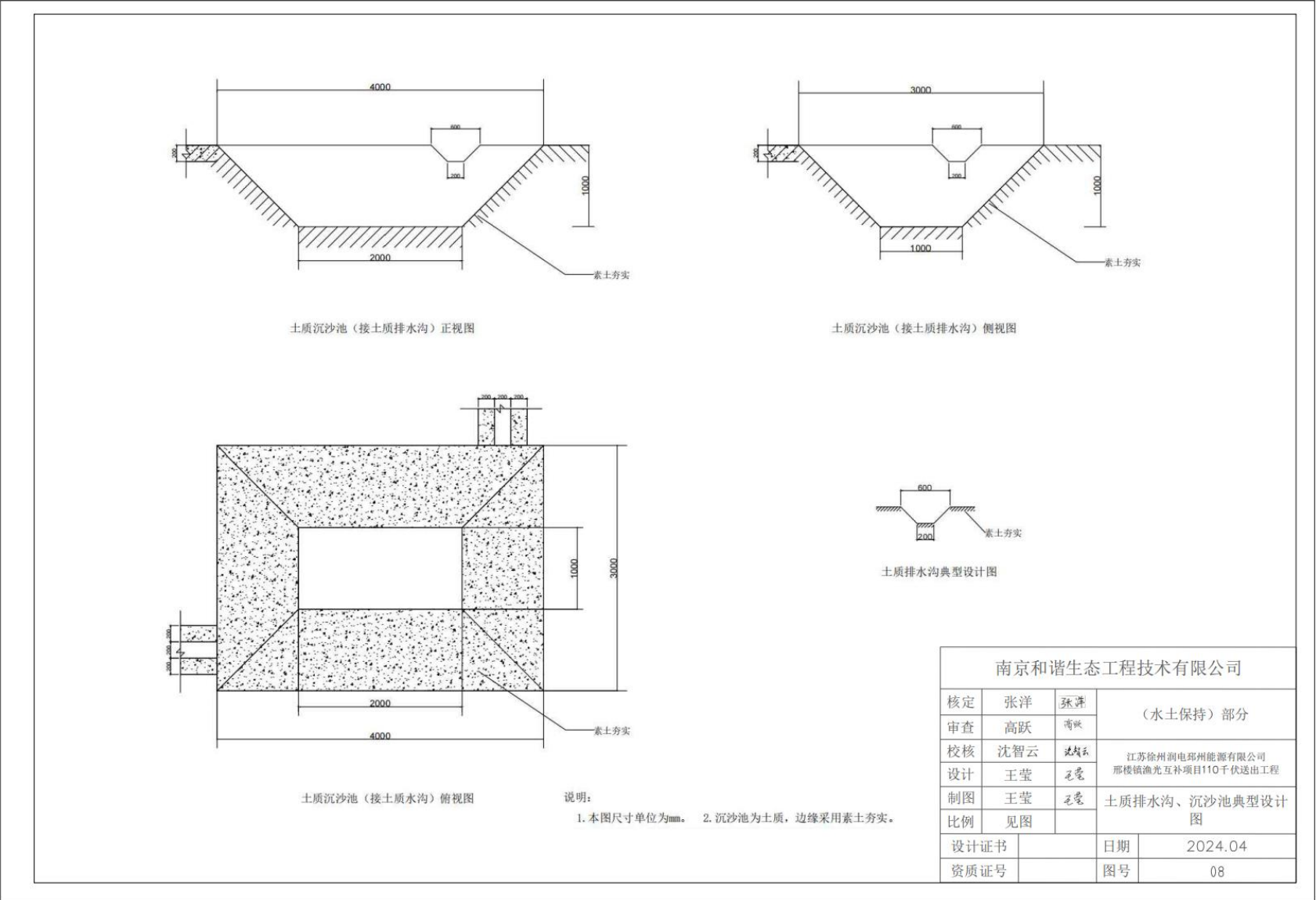
附图 8 临时排水沟、沉沙池典型设计图
