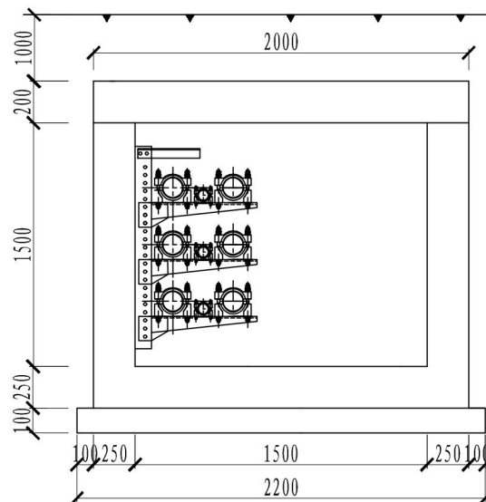
图 1-5 电缆沟断面图
