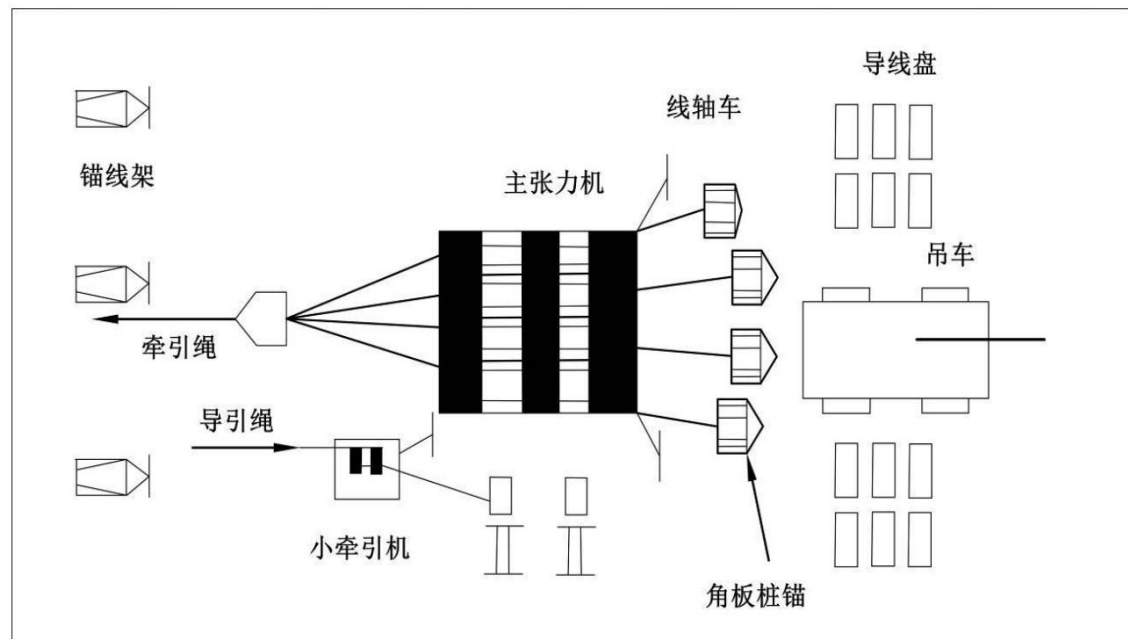
图1-7 张力场布置示意图
