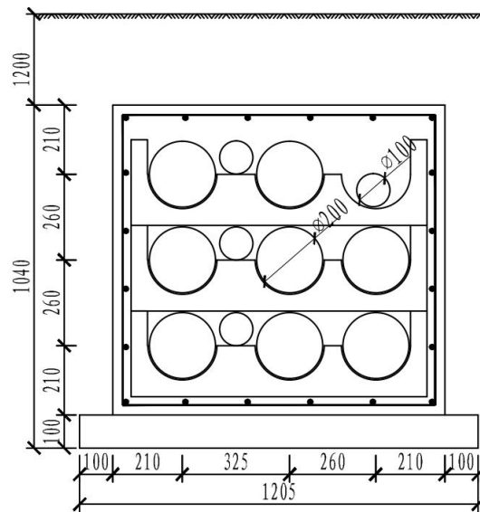
图 1-4 电缆排管断面图
