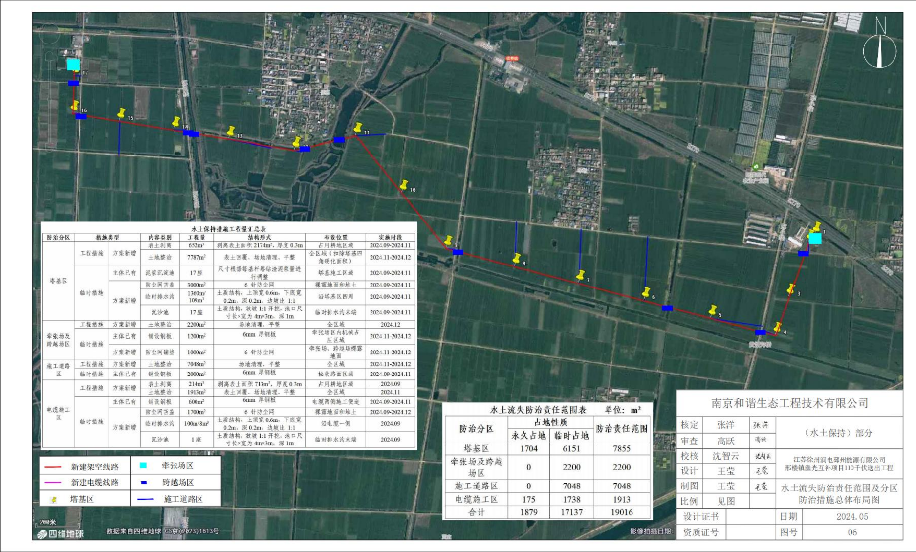
附图 6 水土流失防治责任范围及分区防治措施总体布局图
