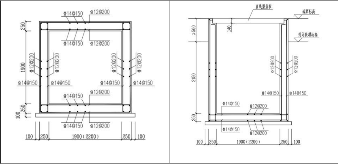
图 1.1-4 1#直线井、2#直线井、中间接头井、三通井、四通井、转角井土建断面图
