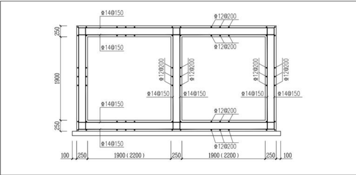
图 1.1-6 双拼直线井、进站双拼电缆井土建断面图
