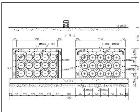
图 1.1-11 2×3×5 φ 200+2×4 φ 100 排管 (加固型)
