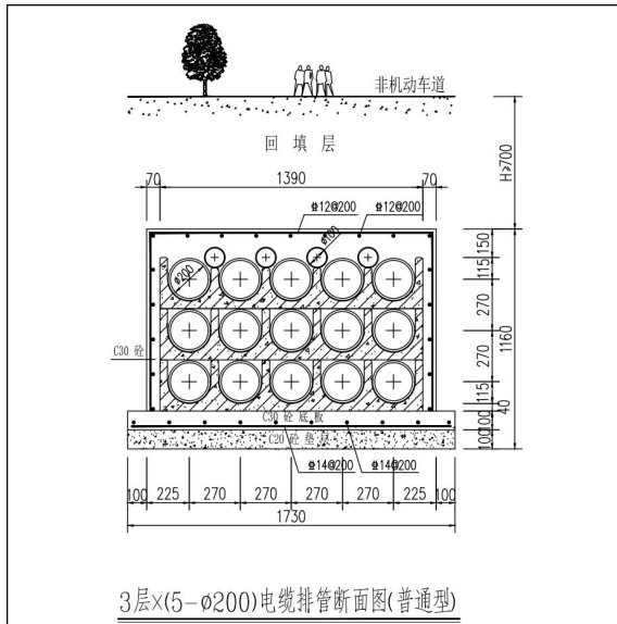
图 1.1-7 3×5 φ 200+4 φ 100 排管 (普通型)
