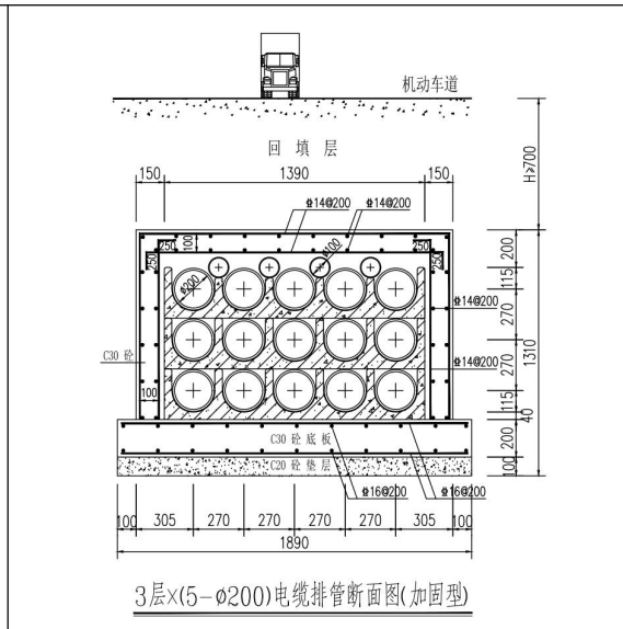
图 1.1-8 3×5 φ 200+4 φ 100 排管 (加固型)
