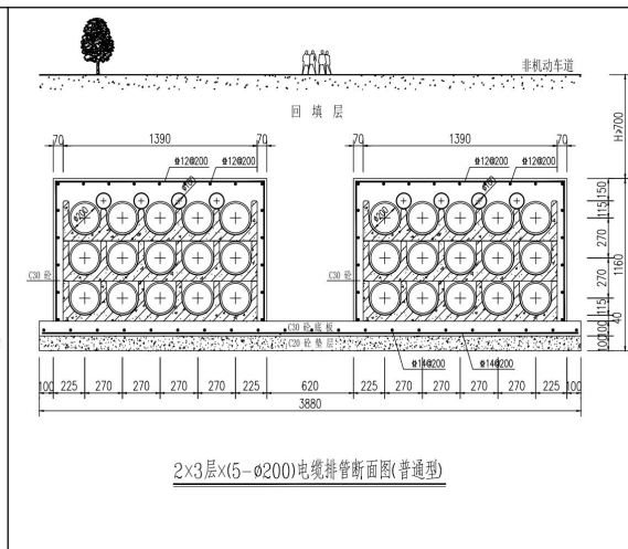
图 1.1-10 2×3×5 φ 200+2×4 φ 100 排管 (普通型)
