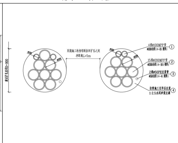
图 1.1-12 15 φ 200+4 φ 100 拉管
