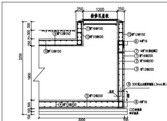
图 1.1-6 转角井断面图
