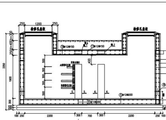
图 1.1-7 预留井断面图
