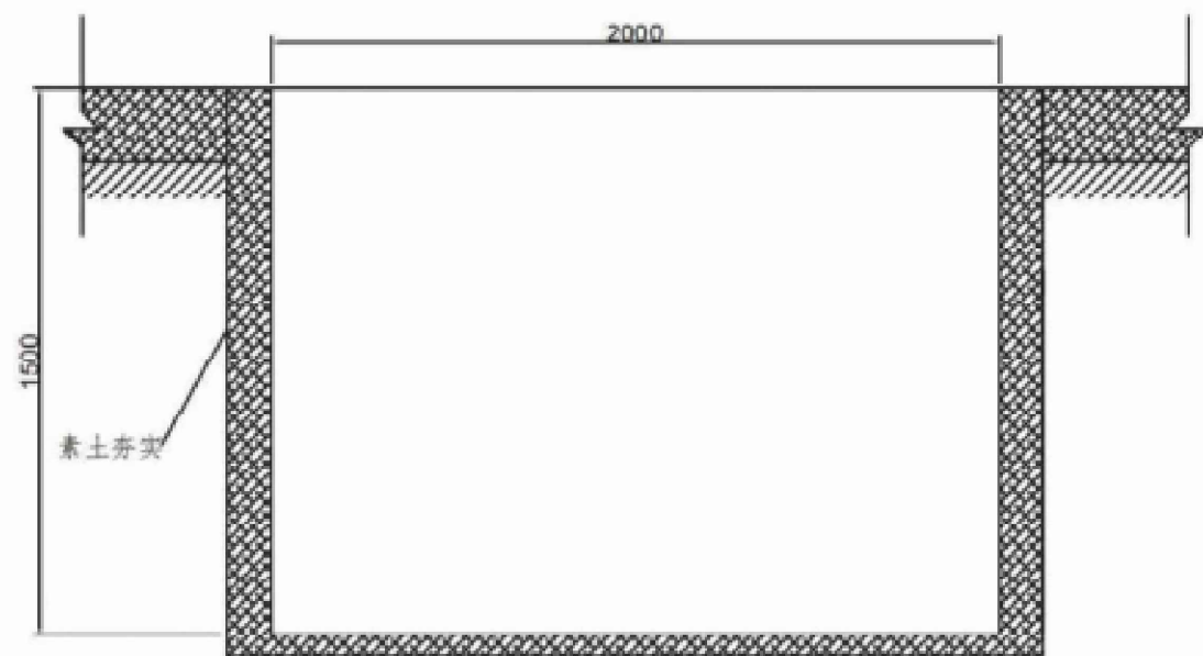
土质沉沙池（接土质排水沟）正视图
