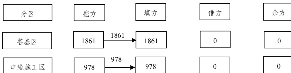
图 1.1-8 土石方平衡框图 单位: m 3
