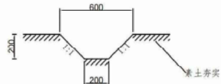
土质排水沟典型设计图
