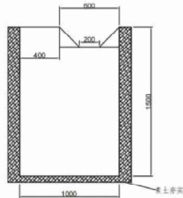
土质沉沙池（接土质排水沟）侧视图
