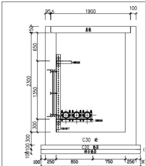
图 1.1-4 电缆沟断面图
