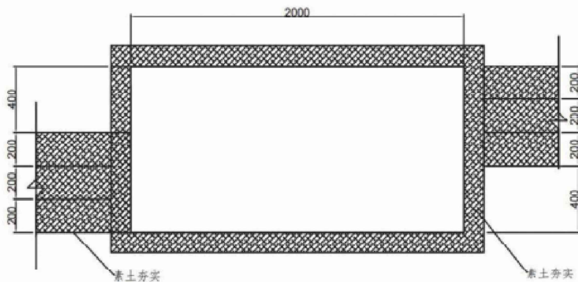
土质沉沙池（接土质排水沟）俯视图
