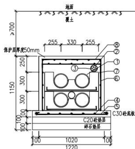
图 1.1-5 电缆排管断面图
