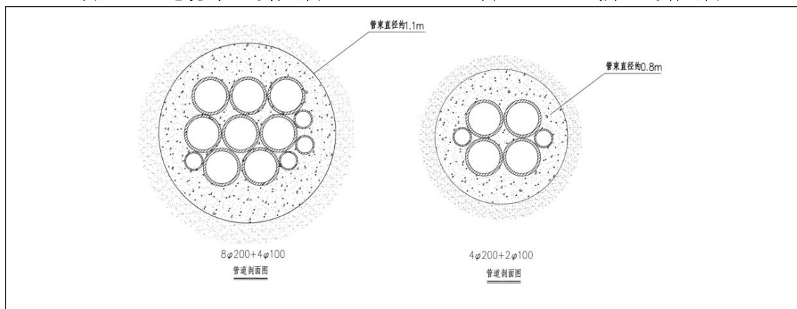
图 1.1-10 排管土建断面图
