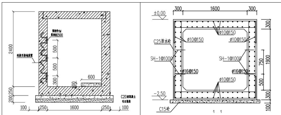
图 1.1-8 电缆沟土建断面图
