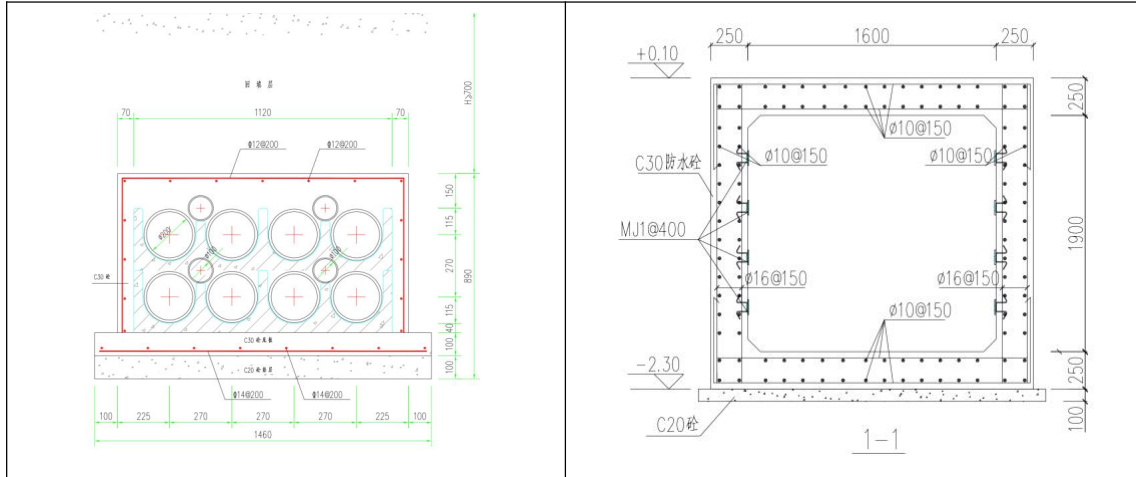
图 1.1-4 排管土建断面图
