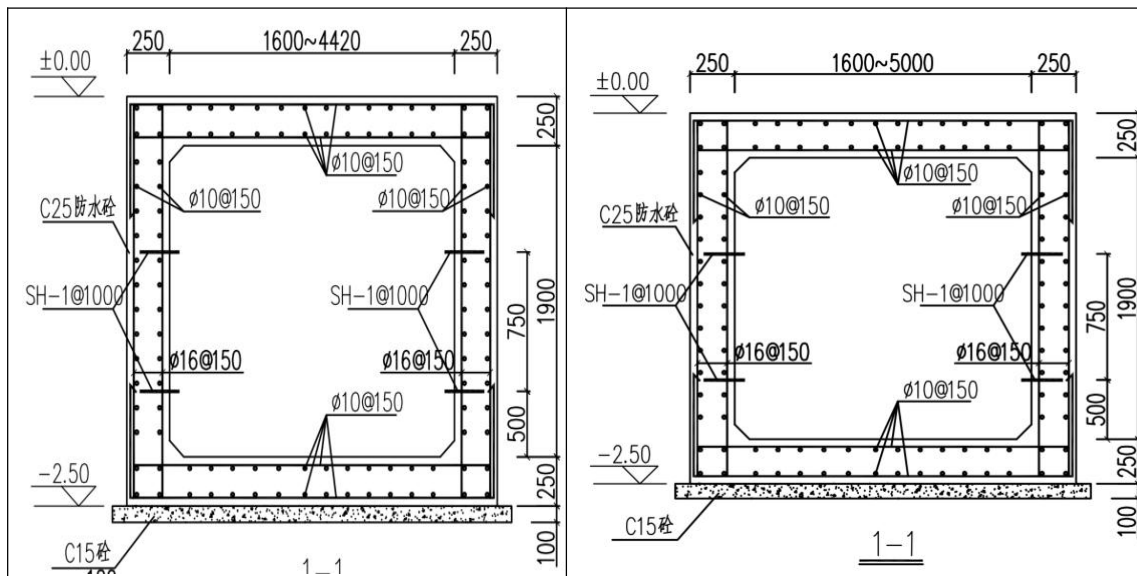
图 1.1-6 三通井土建断面图
