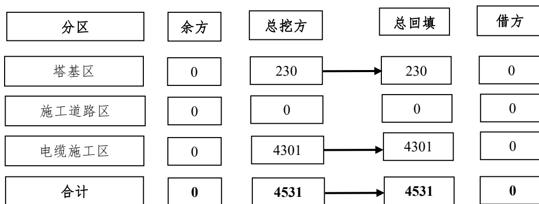
图 1.1-7 土石方平衡流向框图 单位：m 3
