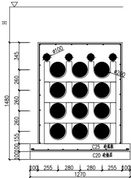
图 1.1-4 排管土建断面图
