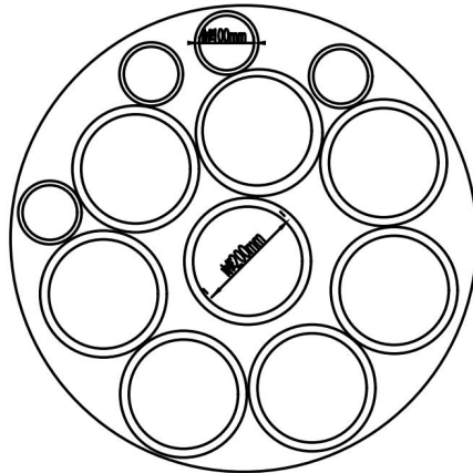
图 1.1-6 拉管土建断面图
