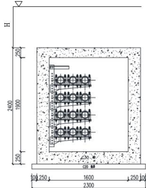
图 1.1-5 电缆沟（井）土建断面图
