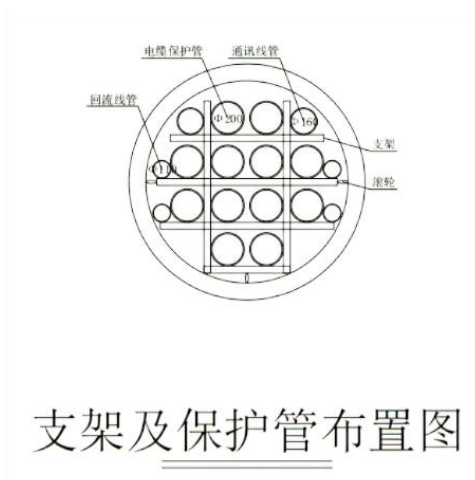
图 1.4-4 顶管断面图
