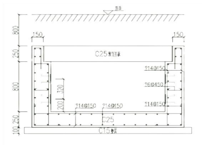
图 1.4-2 电缆沟断面图
