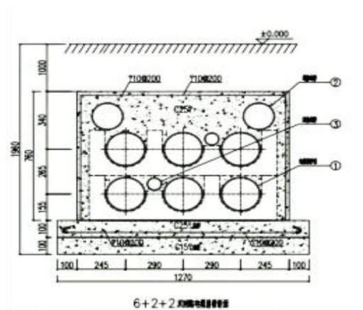
图 1.4-3 排管断面图
