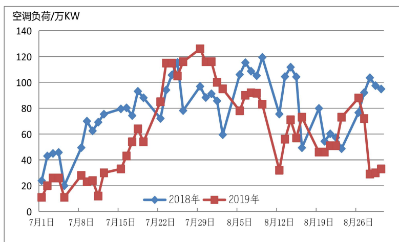
图 2：2018-2019 年夏季日最高空调负荷走势
