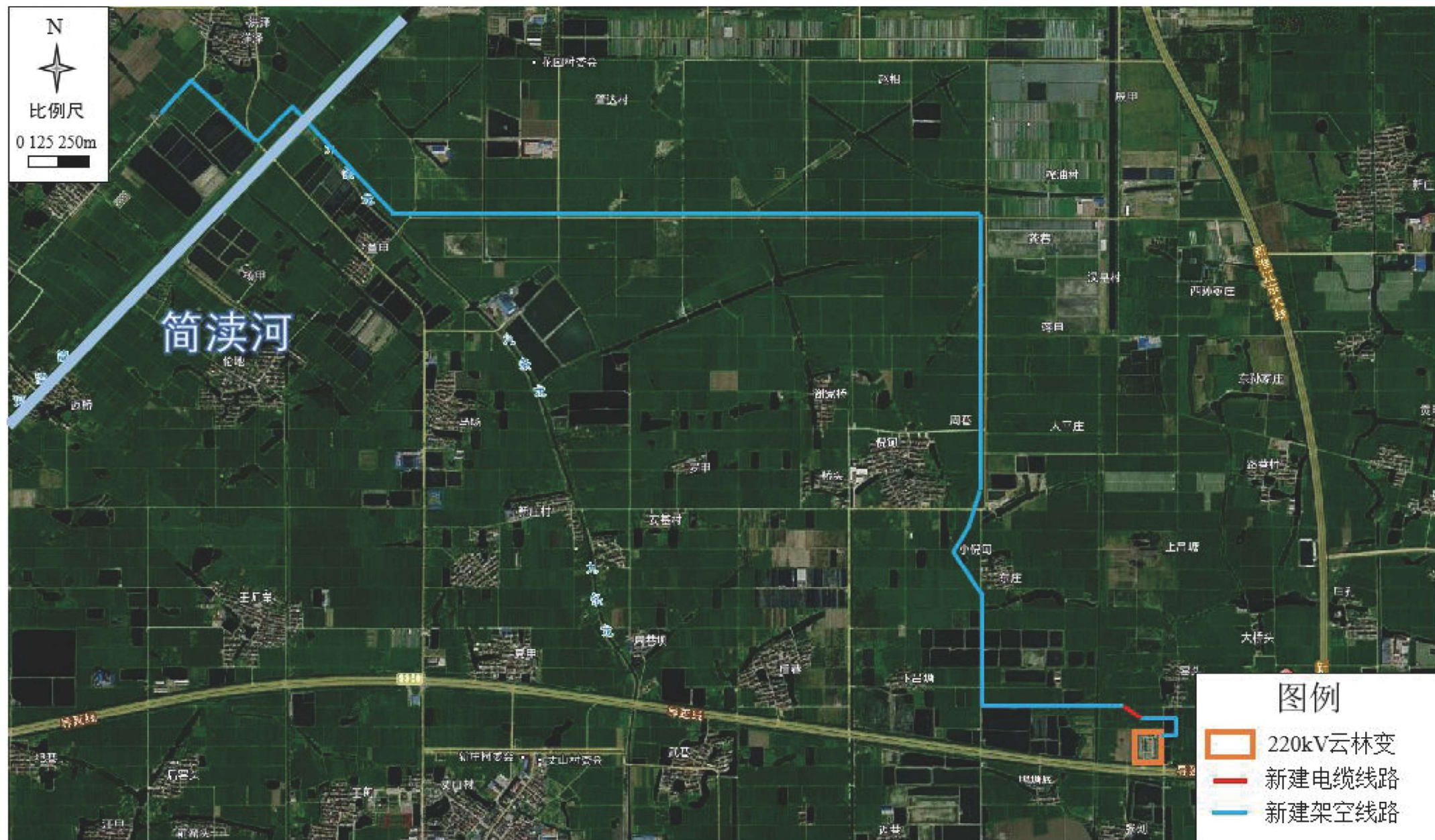
附图2 线路路径图
