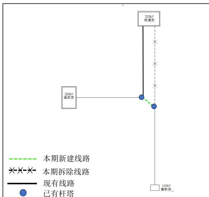
图 1 本项目接线示意图
