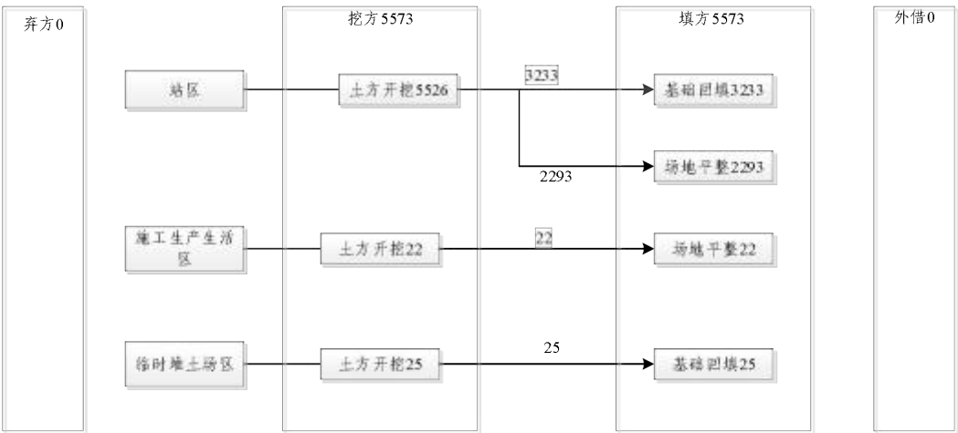
图 1.5-1 工程土方平衡图 单位：m 3
