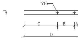
两眼角钢制造尺寸 (毫米)
