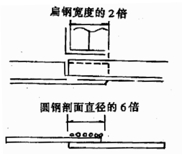
图 3 焊接时搭接长度要求
