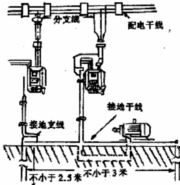
图 2 接地线与接地体示意图
