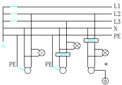
单相（单极或双极）TN-S
