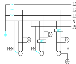
单相（单极或双极）TN-S
