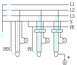
三相（四线，三极或四极）TN-S
