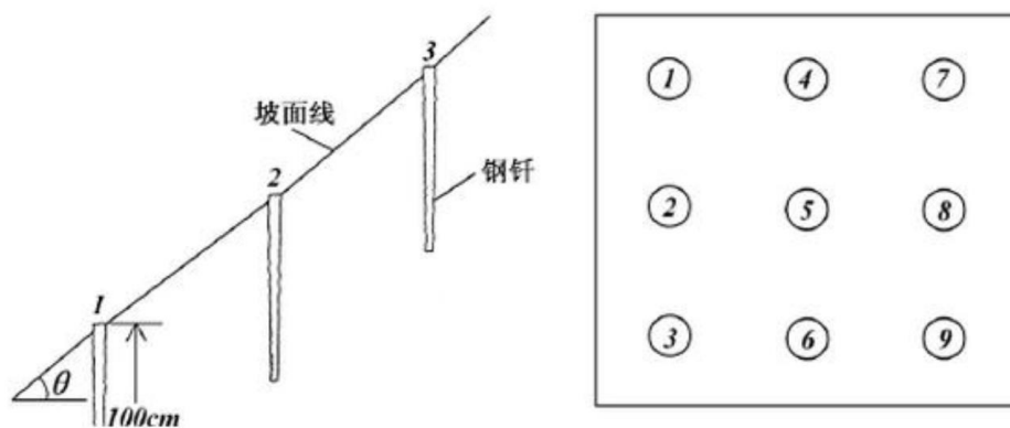
图 3-1 水土流失简易观测场示意图
