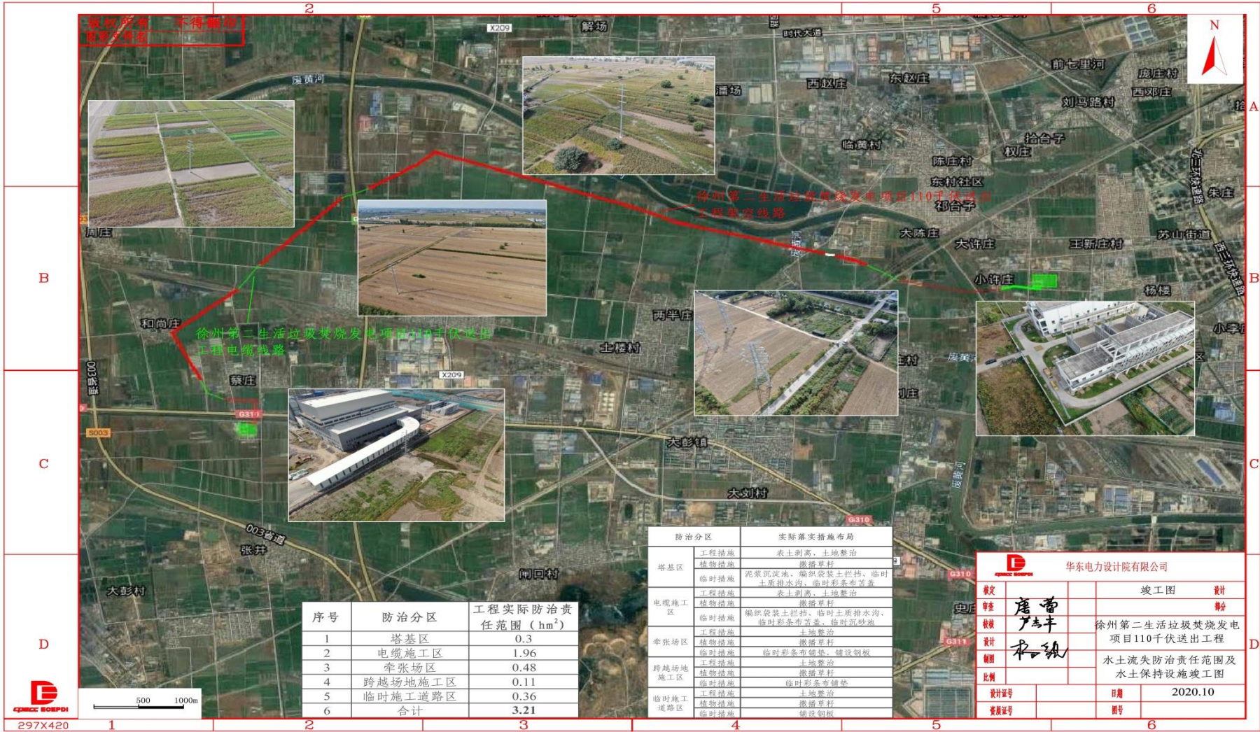
(2) 水土流失防治责任范围及水土保持措施布设竣工图
