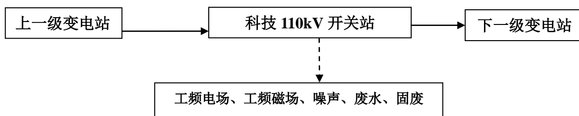
图 1 江苏常州科技 110kV 开关站新建工程工艺流程及产污环节示意图
