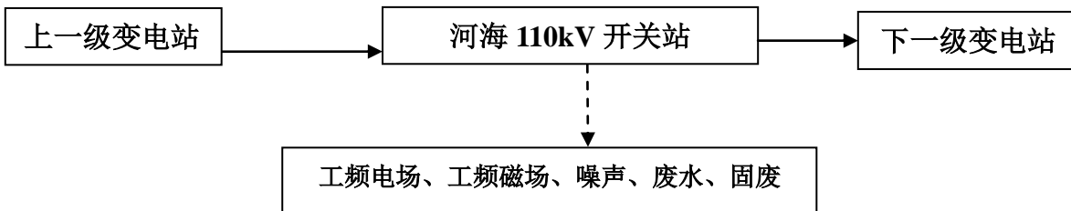
图 1 江苏常州河海 110kV 开关站新建工程工艺流程及产污环节示意图
