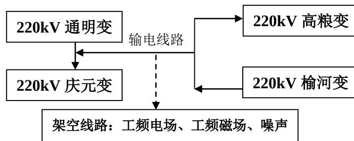
图 1 盐城高粮/榆河~通明 220 千伏线路工程工艺流程及产污环节示意图
