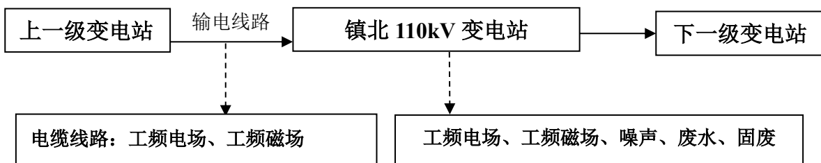
图 1 江苏常州镇北 110kV 输变电工程工艺流程及产污环节示意图
