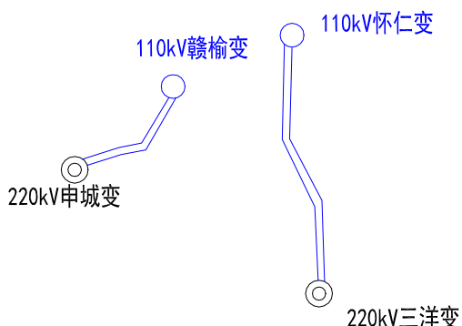
图 1-1 本工程实施前系统接线图
