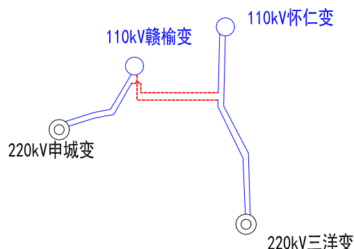
图 1-2 本工程实施后系统接线图
