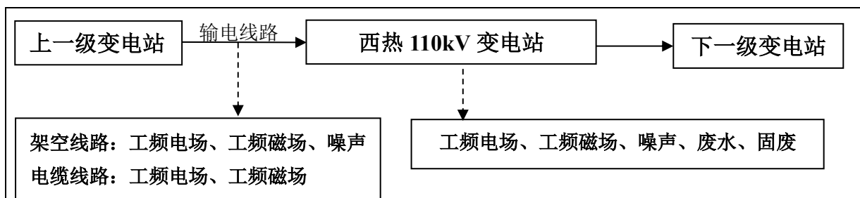
图 1 南通西热 110kV 输变电工程工艺流程及产污环节示意图
