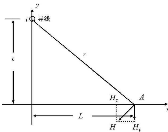
图 3.2-4 磁场向量图
