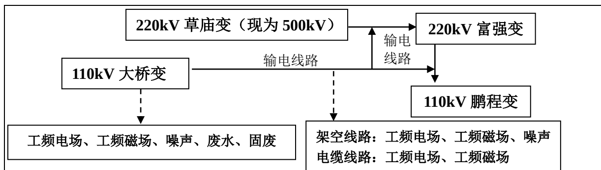
图 2 江苏盐城大桥 110 千伏输变电工程工艺流程及产污环节示意图 污染分析：
