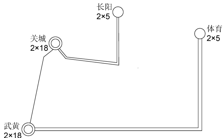
图 1-1 接入系统方案图（改接前）
