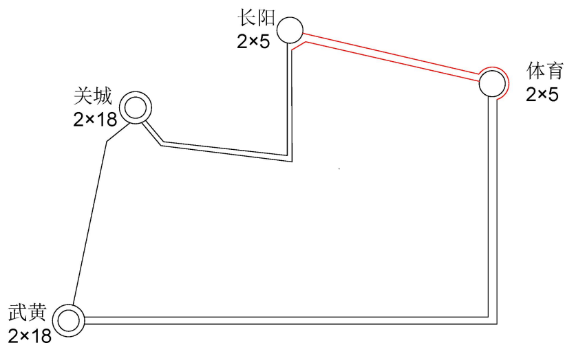
图 1-2 接入系统方案图（改接后）
