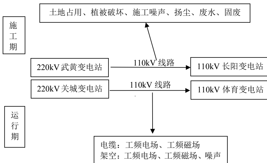
图 5-1 输电线路工艺流程及主要产污环节示意图
