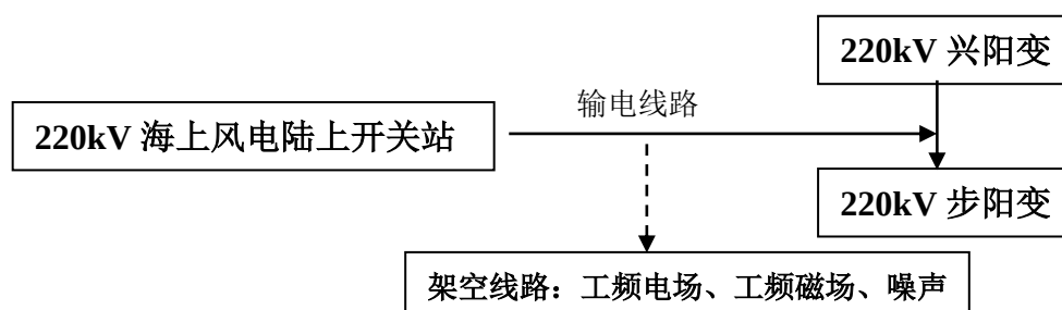
图1 江苏盐城射阳龙源海上南区 H2#风电 220kV 送出工程工艺流程及产污环节示意图
