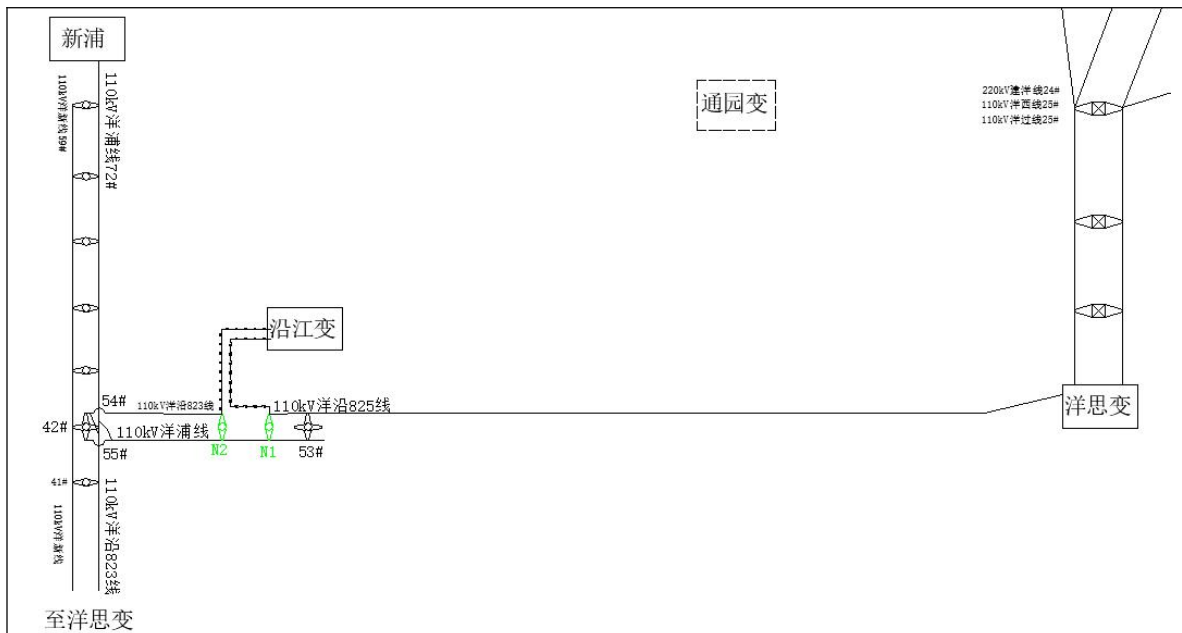
图 1-1 沿江～通园、洋思～通园、洋思～新浦 110kV 线路工程实施前系统接线图
