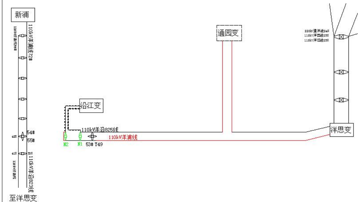
图 1-2 沿江～通园、洋思～通园、洋思～新浦 110kV 线路工程实施后系统接线图
