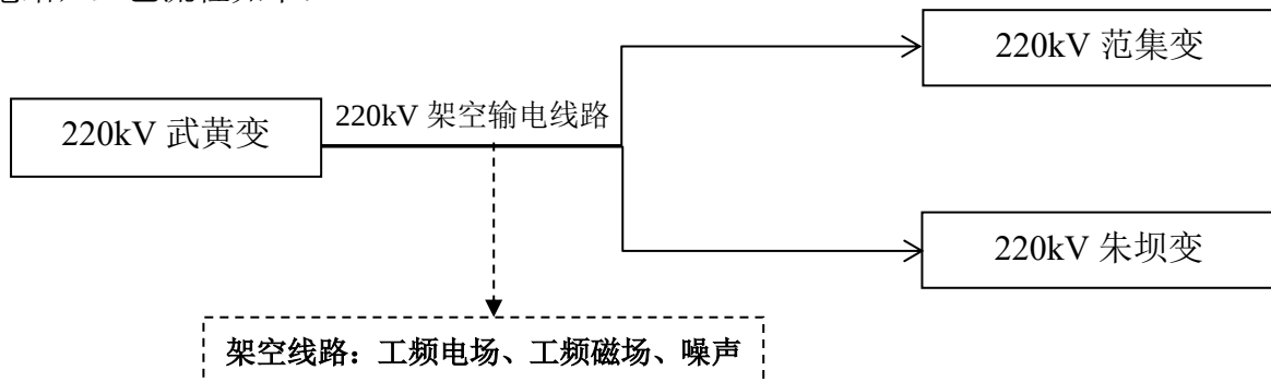
图 1 本输电线路工程工艺流程及产污环节示意图
