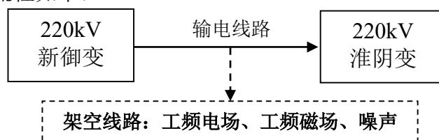
图2 本工程输电线路工程工艺流程及产污环节示意图
