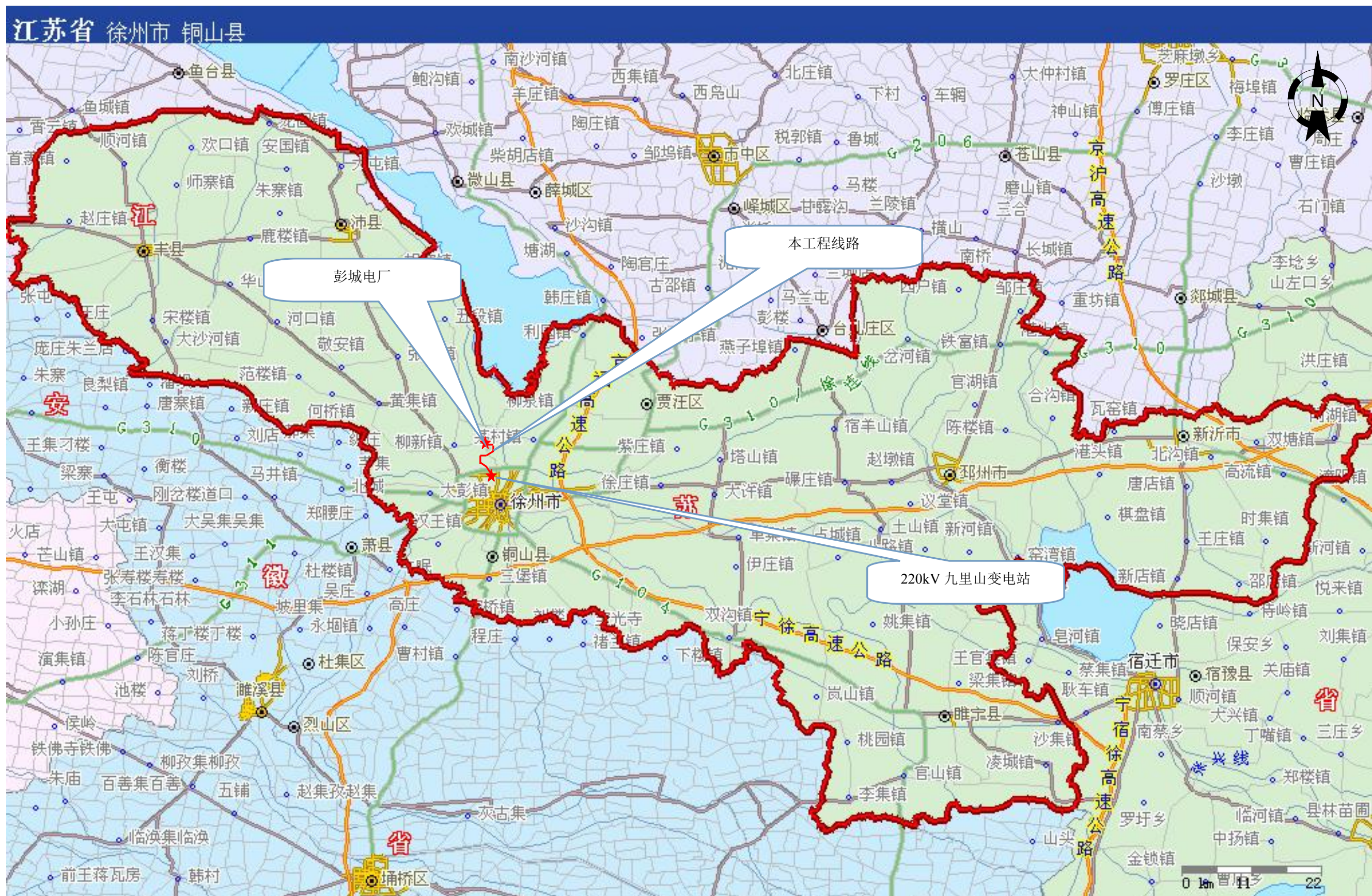
附图 1、江苏徐州彭城电厂至九里山、商圈 220kV 线路改造工程地理位置示意图
