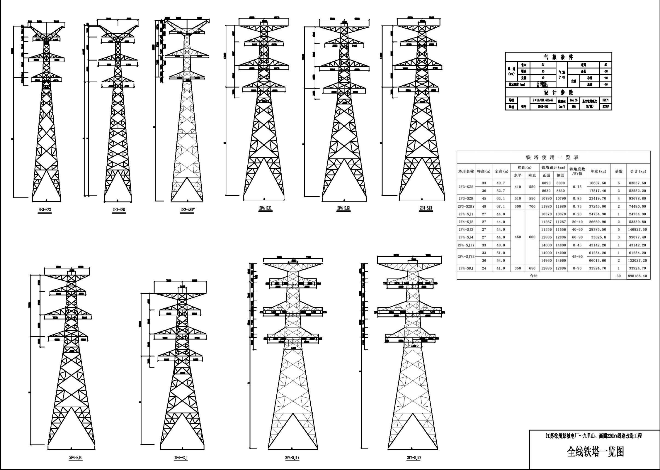
附图 5、江苏徐州彭城电厂至九里山、商圈 220kV 线路改造工程线路杆塔示意图
