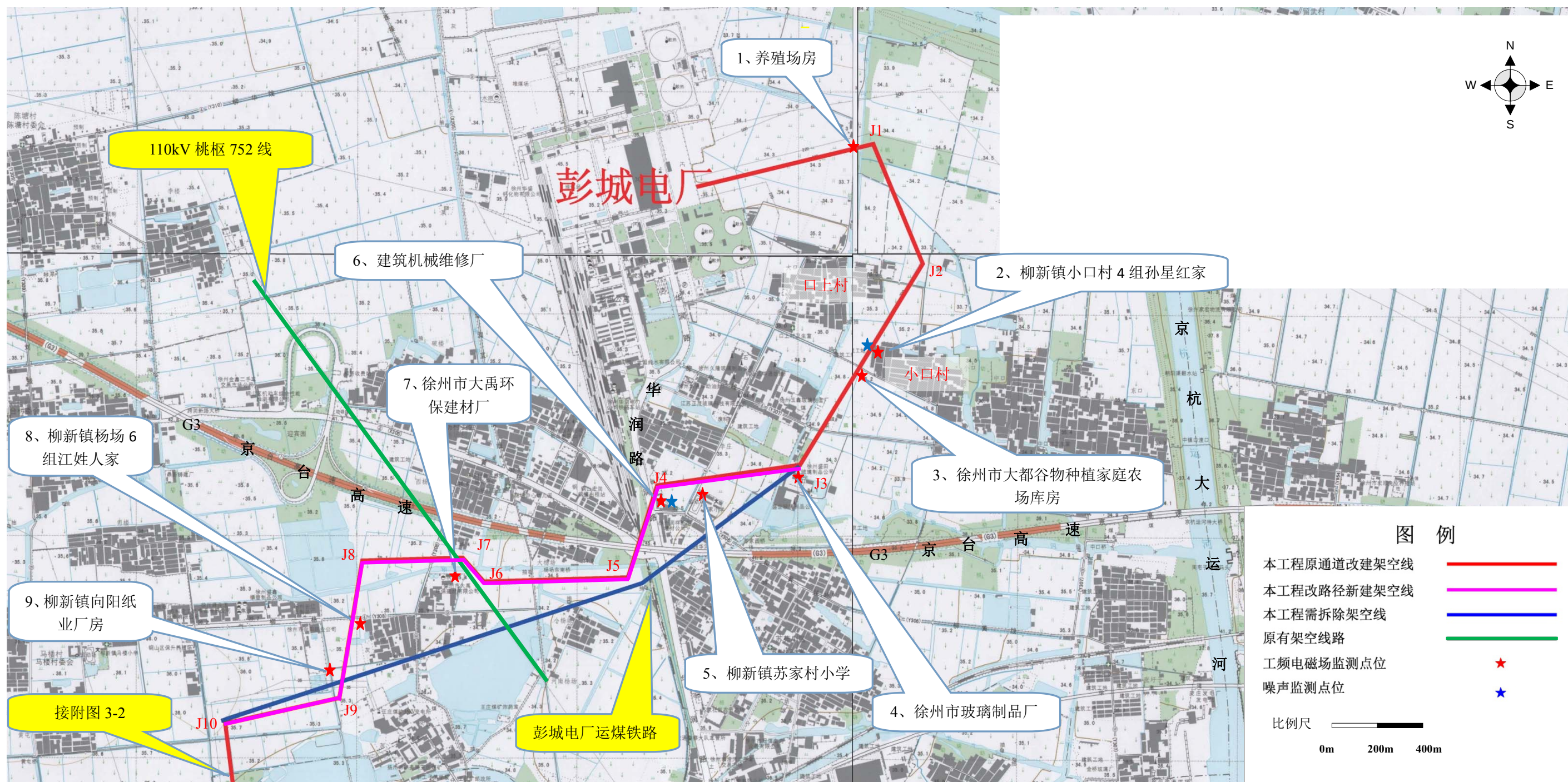
附图 3-1、江苏徐州彭城电厂至九里山、商圈 220kV 线路改造工程线路路径及监测点位示意图
