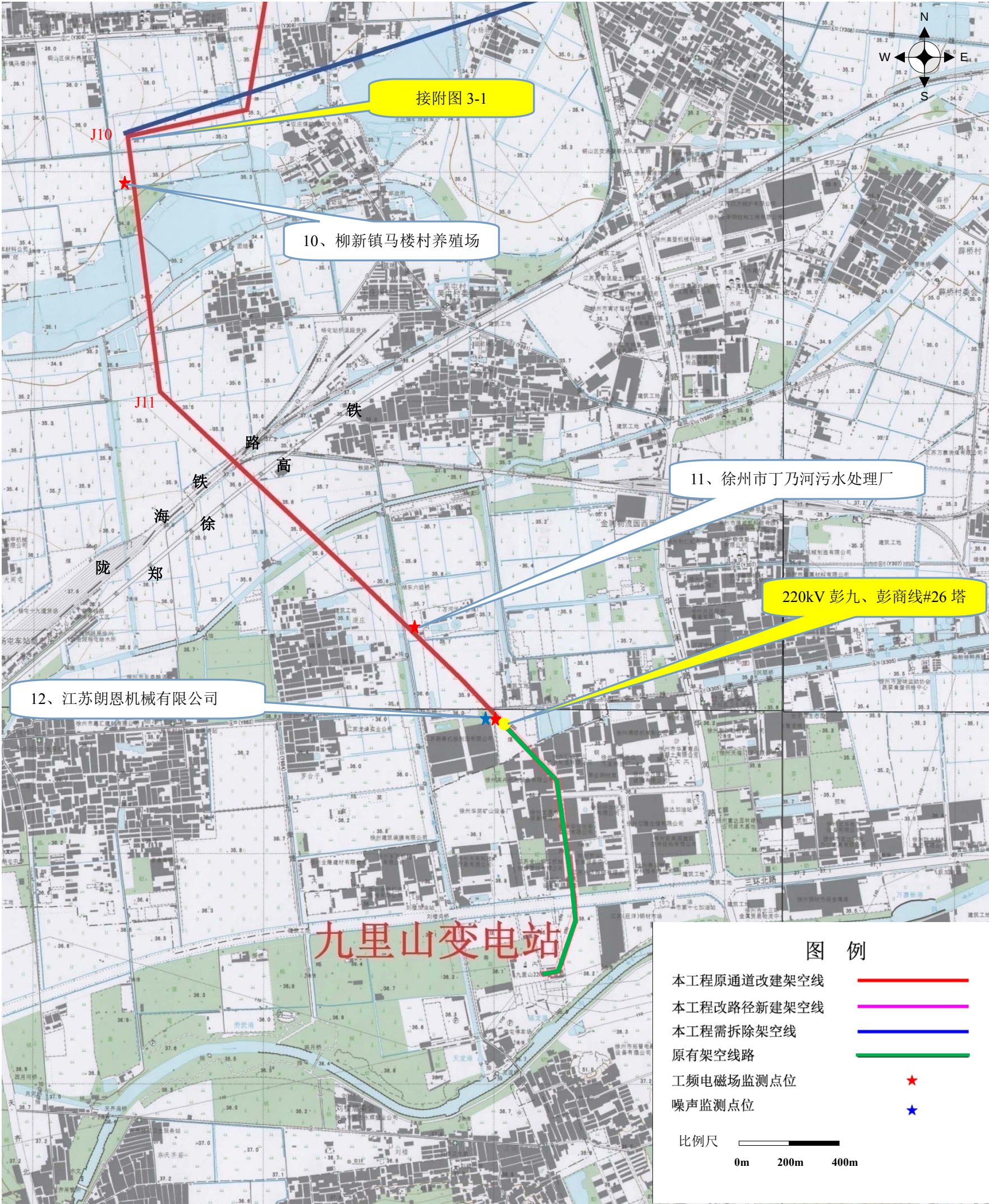
附图 3-2、江苏徐州彭城电厂至九里山、商圈 220kV 线路改造工程线路路径及监测点位示意图
