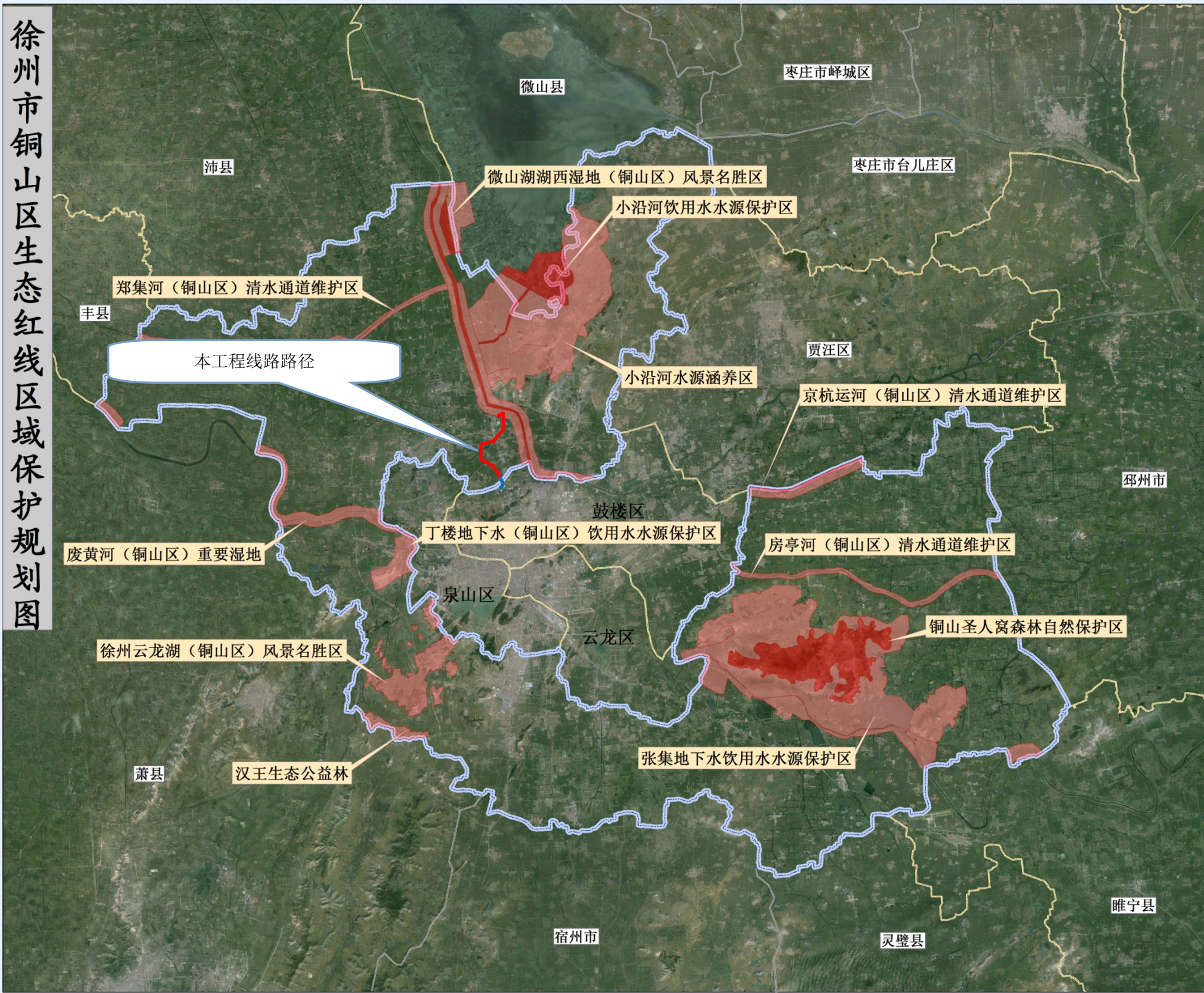
附图2 江苏徐州彭城电厂至九里山、商圈 220kV 线路改造工程生态红线区相对位置关系图
