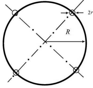
图 3.1-2 电位系数计算图 图 3.1-3 等效半径计算图
