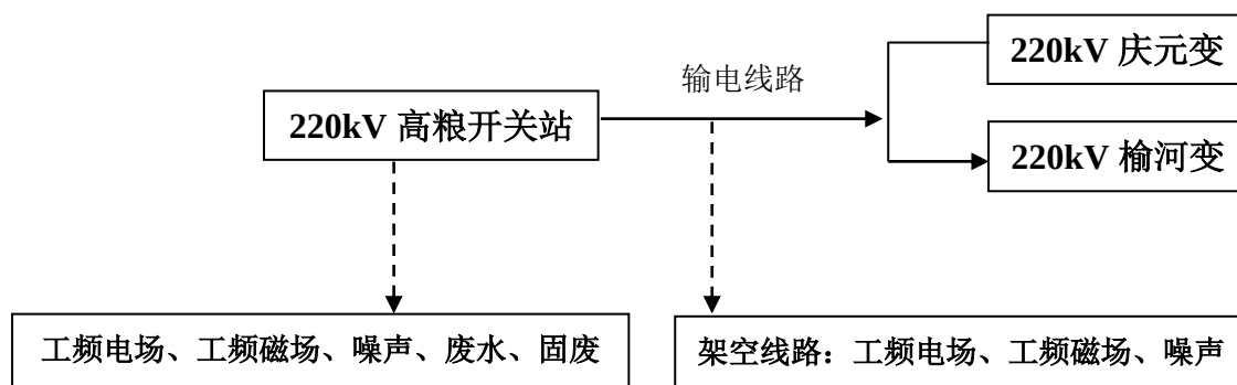
图 1 盐城高粮 220 千伏输变电工程工艺流程及产污环节示意图
