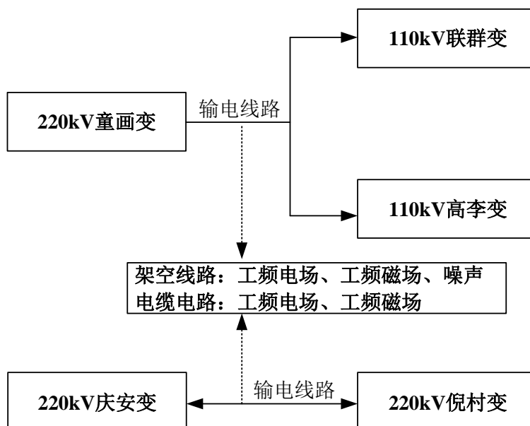
图 1 本工程 110kV 输电线路工艺流程及产污环节示意图
