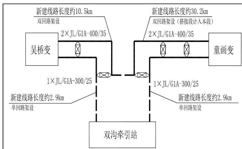
图 1 本工程线路接入方案示意图
