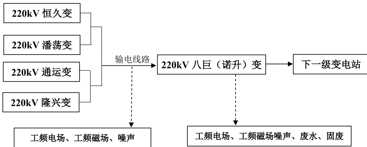
图 1 220kV 输变电工程工艺流程及产污环节示意图
